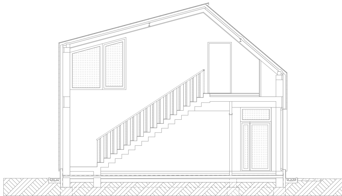
B-B METSZET
