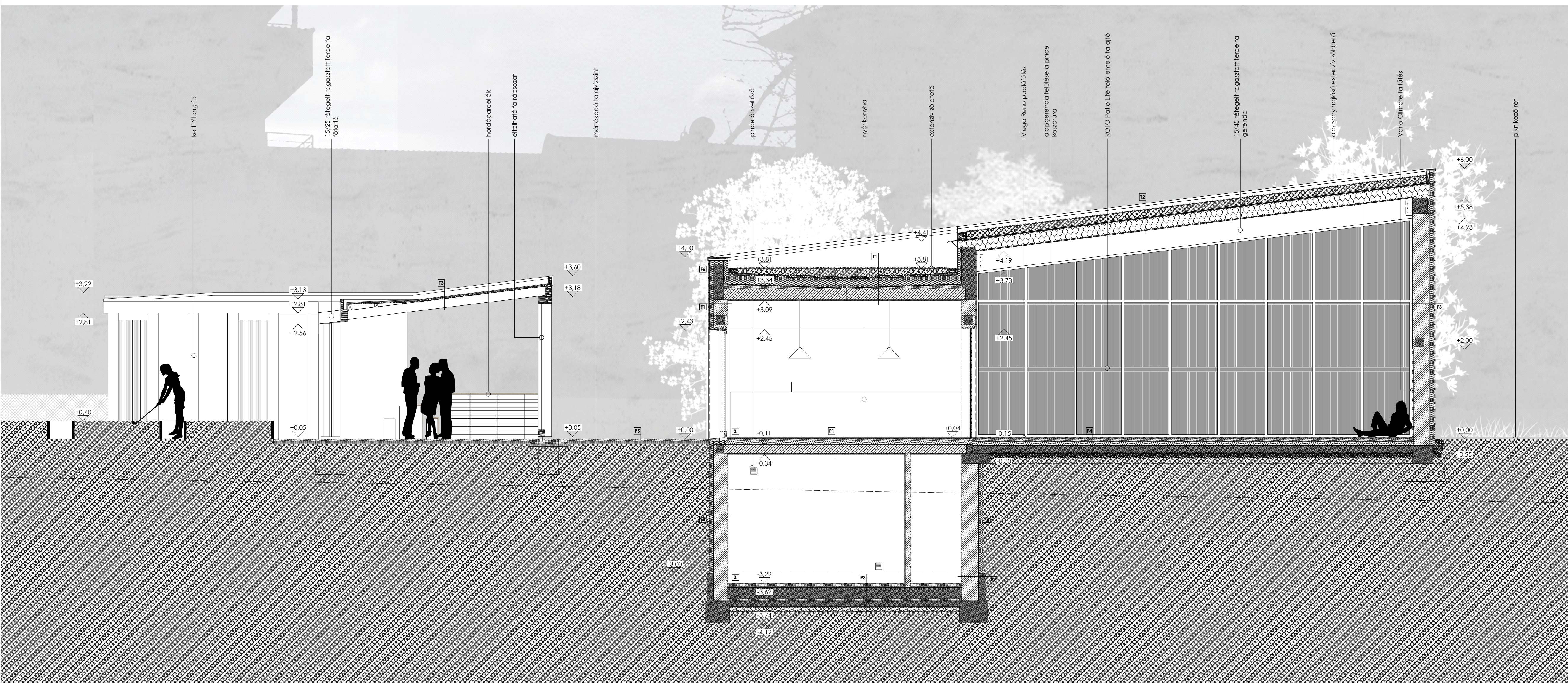
A-A METSZET
