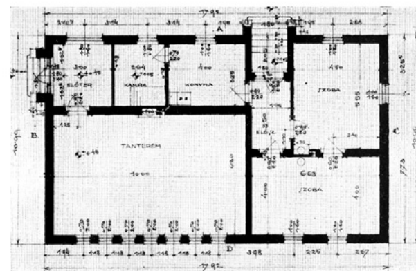
ALAPRAJZ
