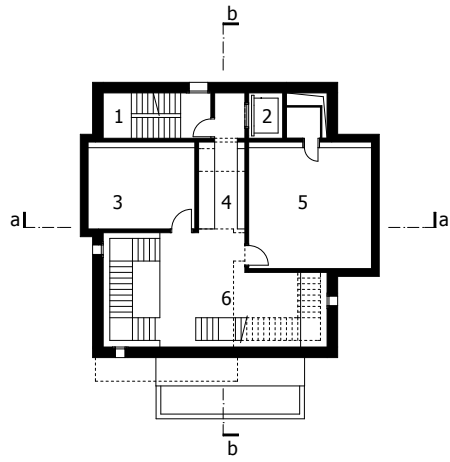
Második emeleti alaprajz - Second floor plan M 1:400 - Scale 1:400
