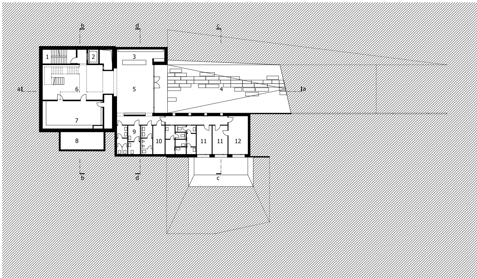
Földszinti alaprajz - Ground floor plan M 1:400 - Scale 1:400
