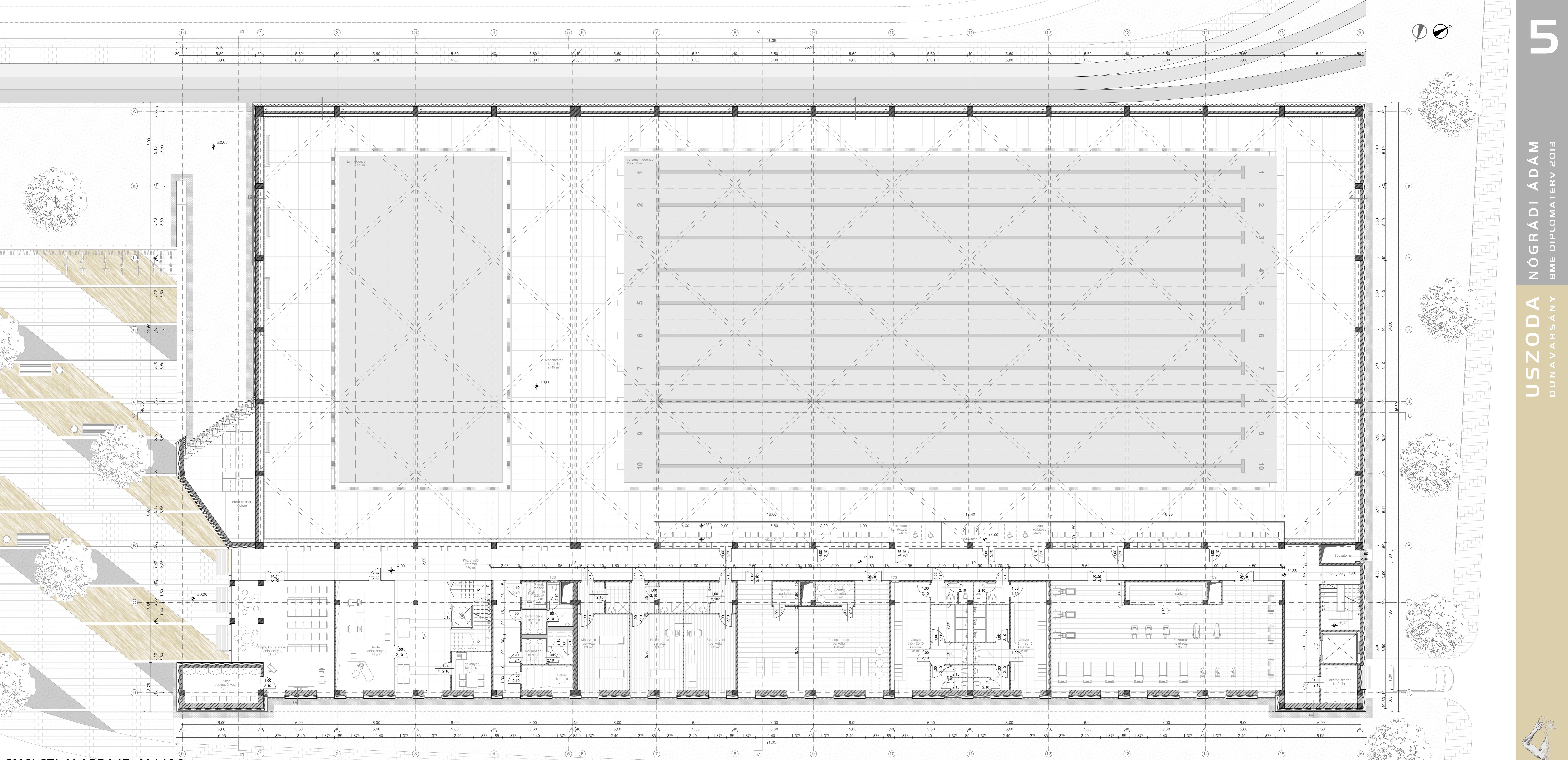
EMELETI ALAPRAJZ M 1:100
