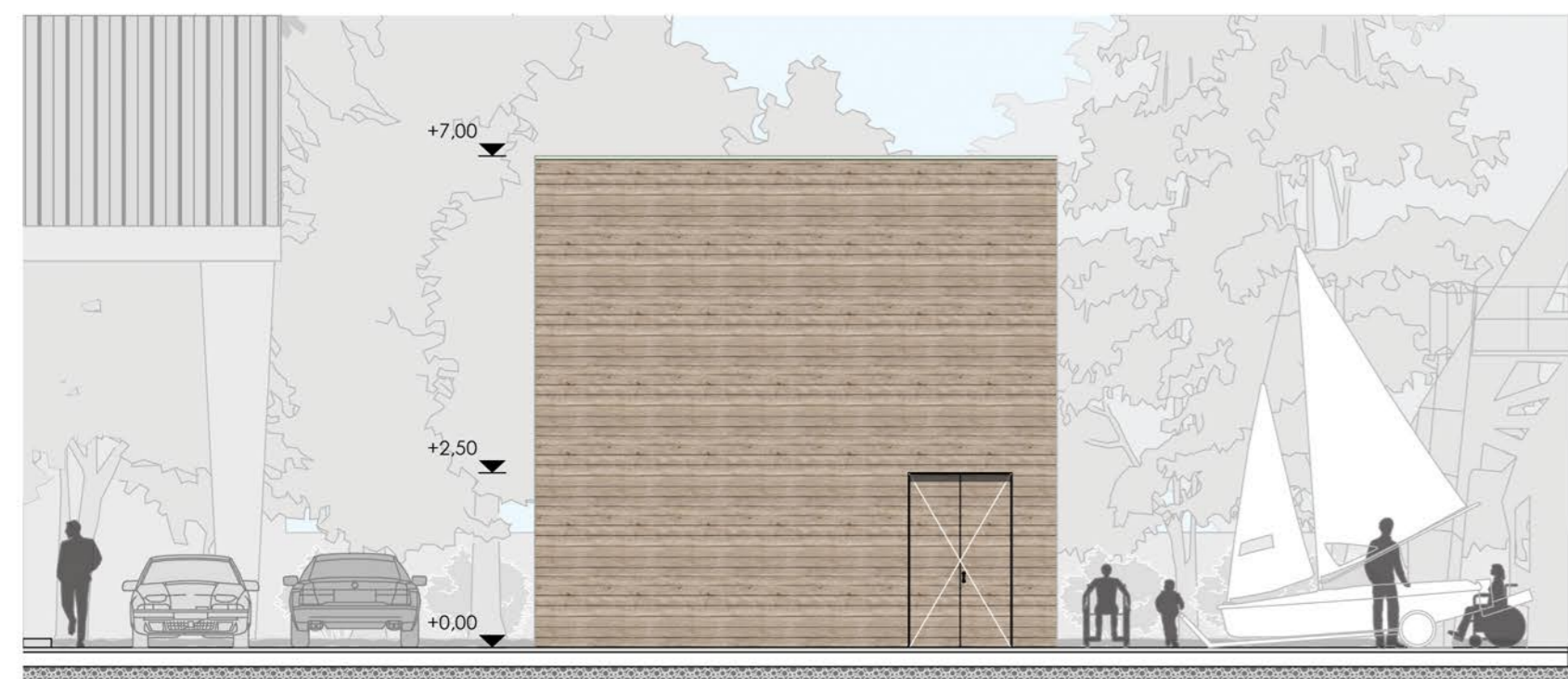
Északkeleti homlokzat
