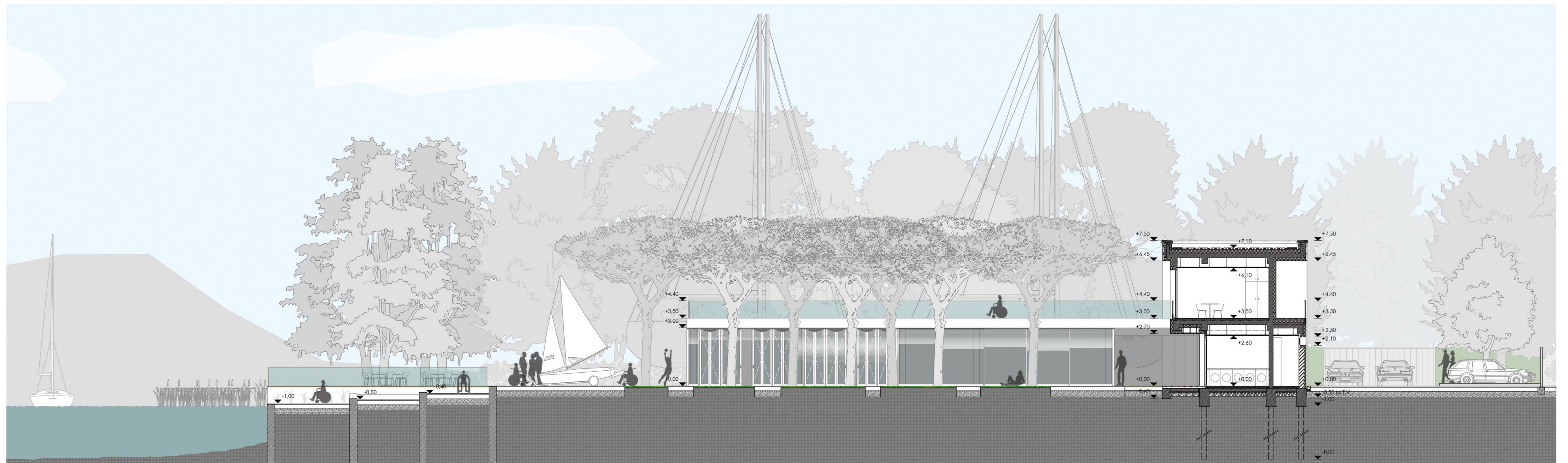
C-C metszet
