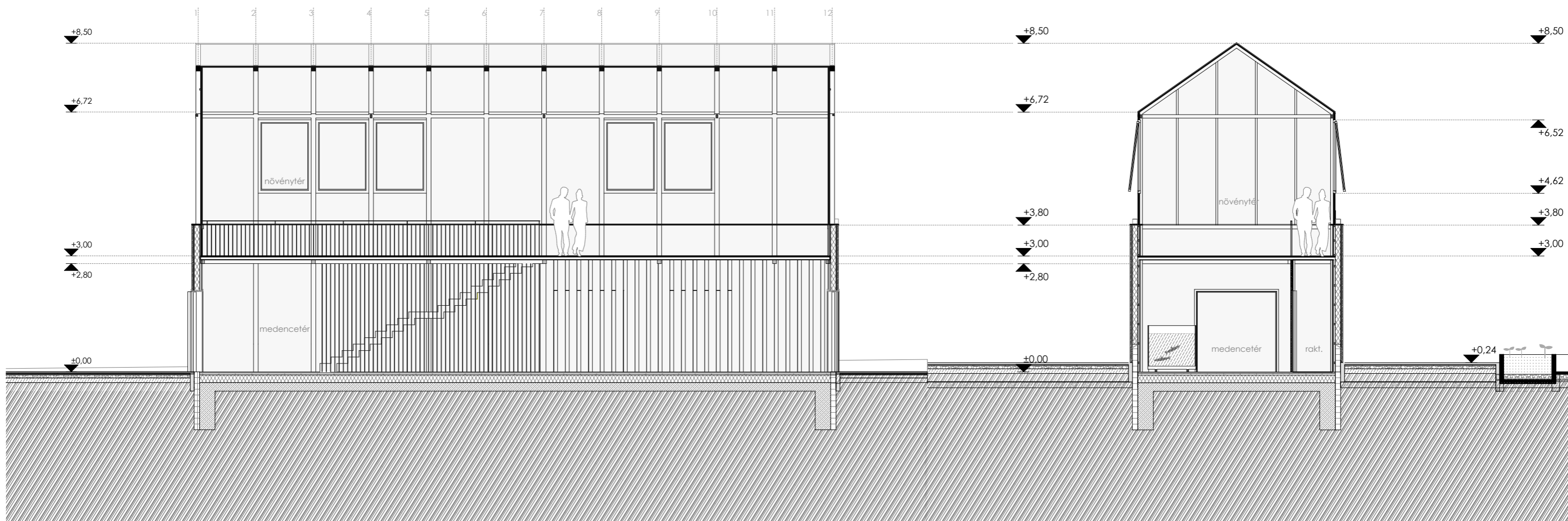
Ü1 metszet üvegház m 1:100
