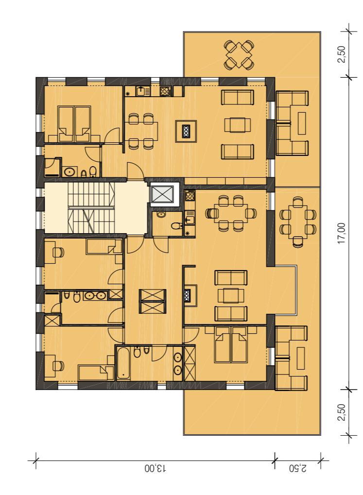
2. OBERGESCHOSS
