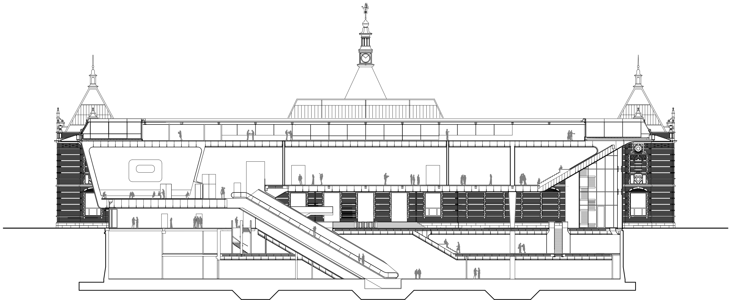
Longitudinal section
