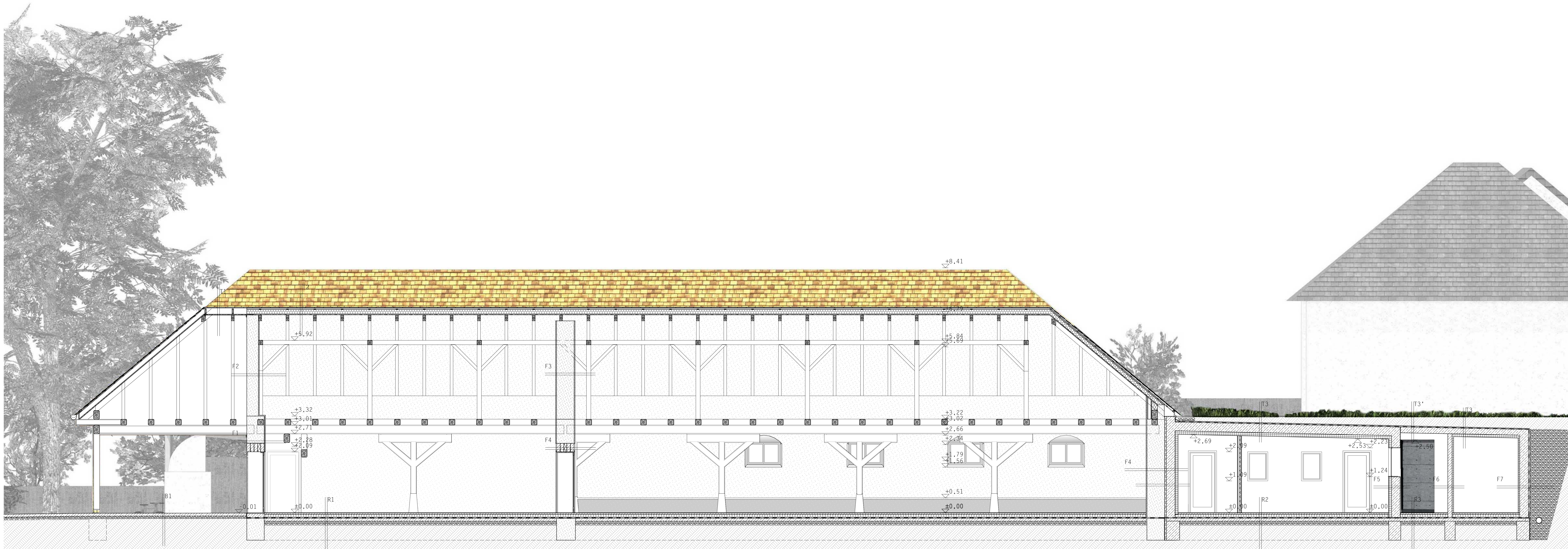
1-1 metszet m1:50
