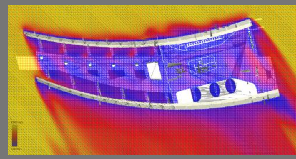
Gravitációs szellőzés szimulációs vizsgálata
