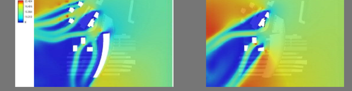
Különböző magasságban végzett széláramlás szimulációk
