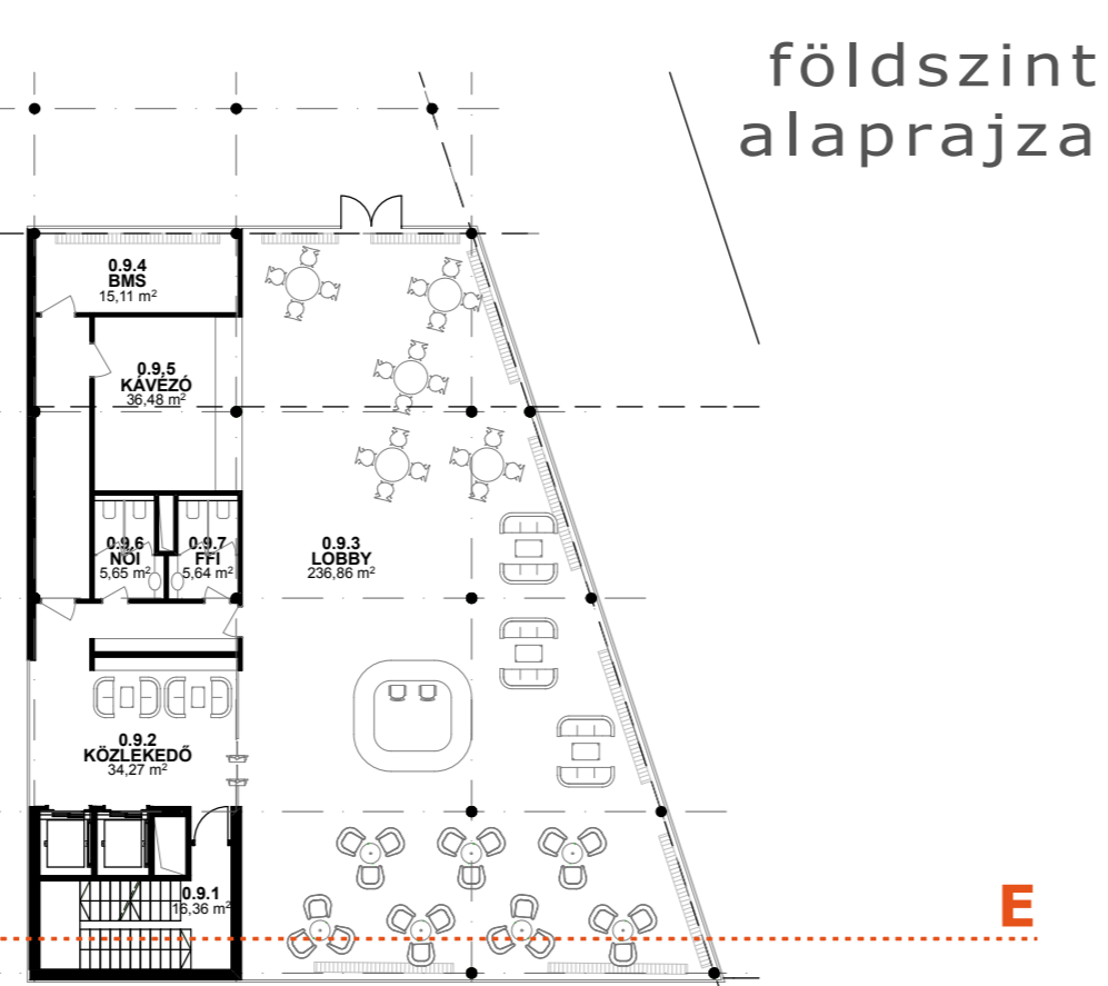
Béirodaház alaprajzai
