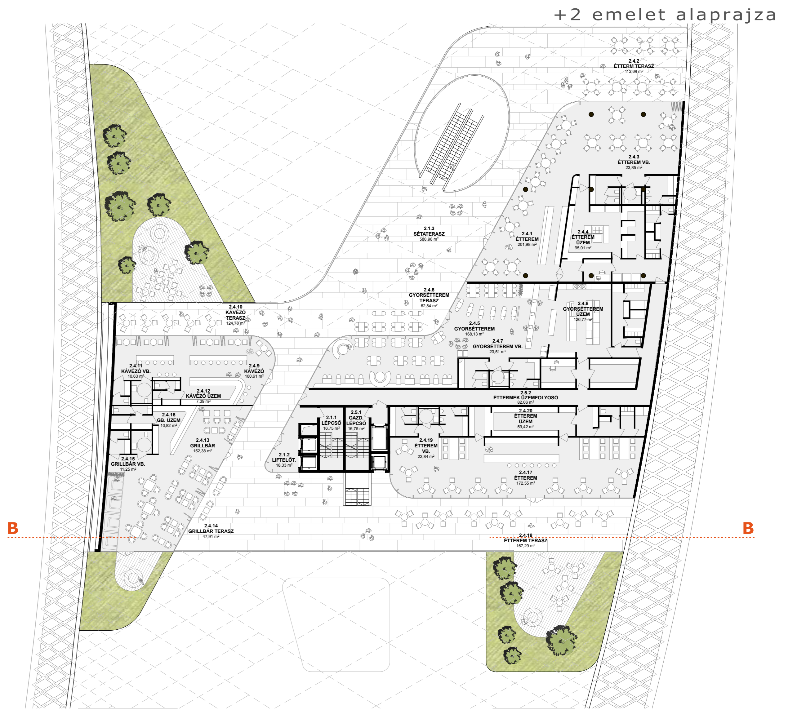
MÁV Irodaház alaprajzai
