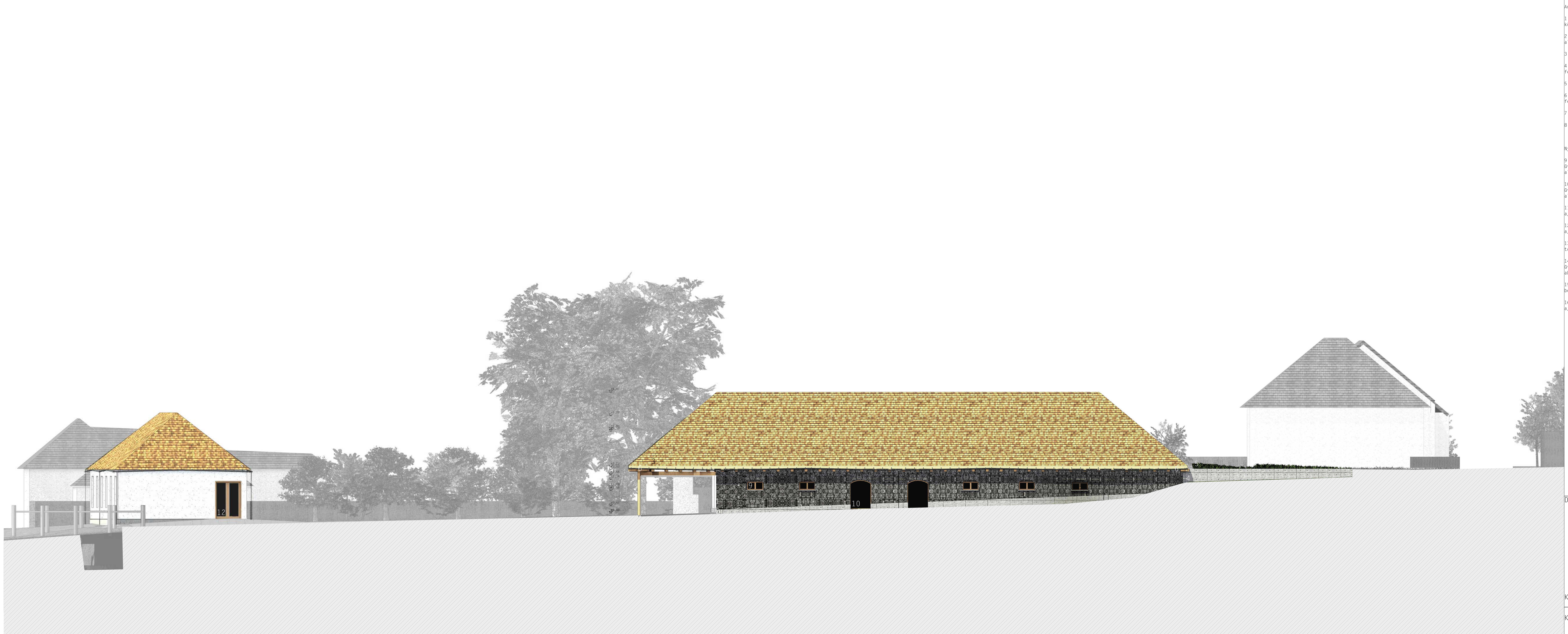
Rendezvényház Déli homlokzat m1:100
