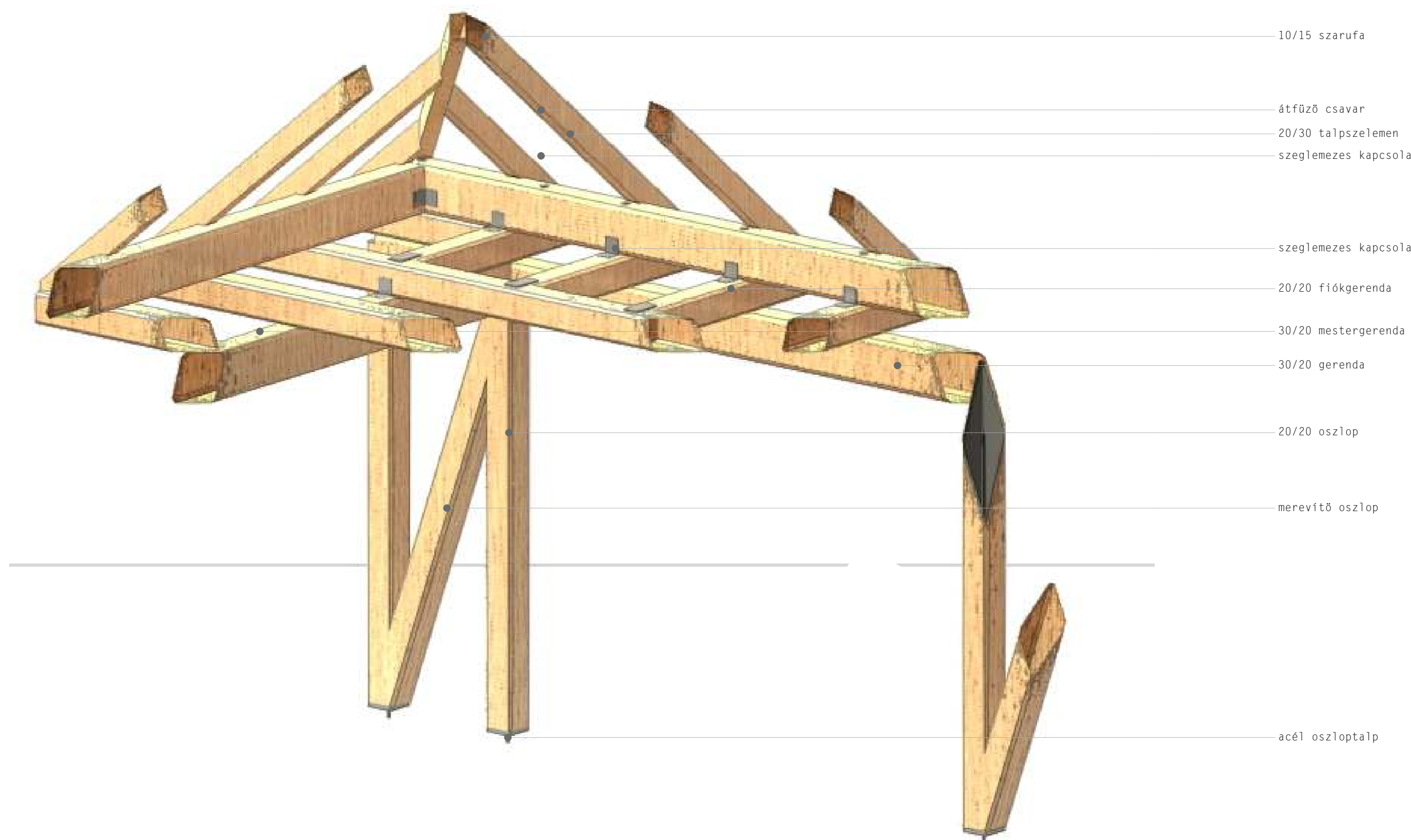
Részletrajzok m1:10
