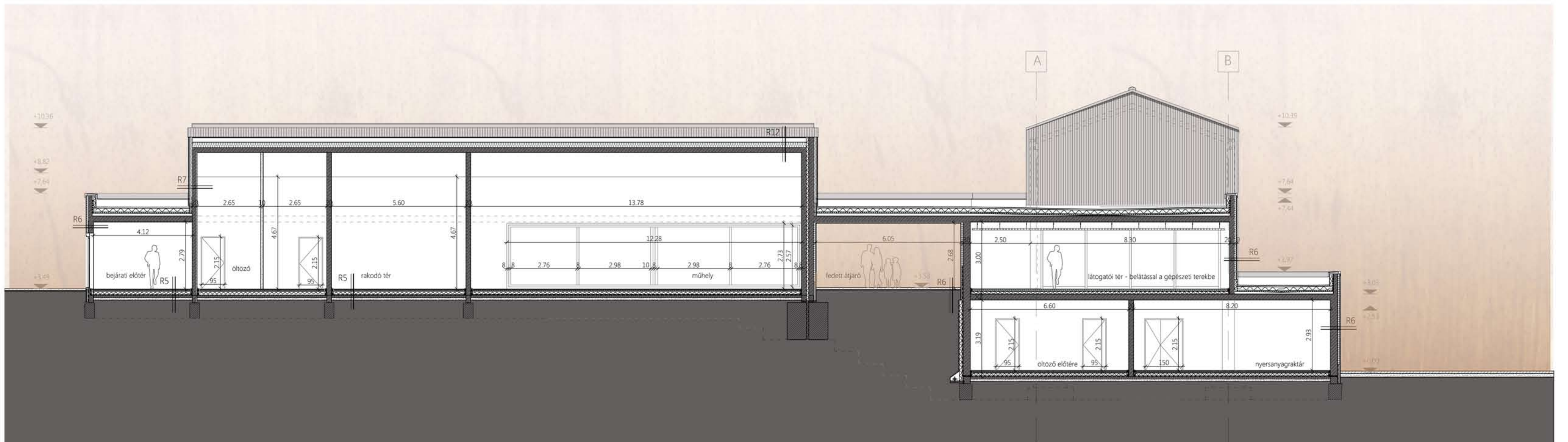
4 - 4 metszet
