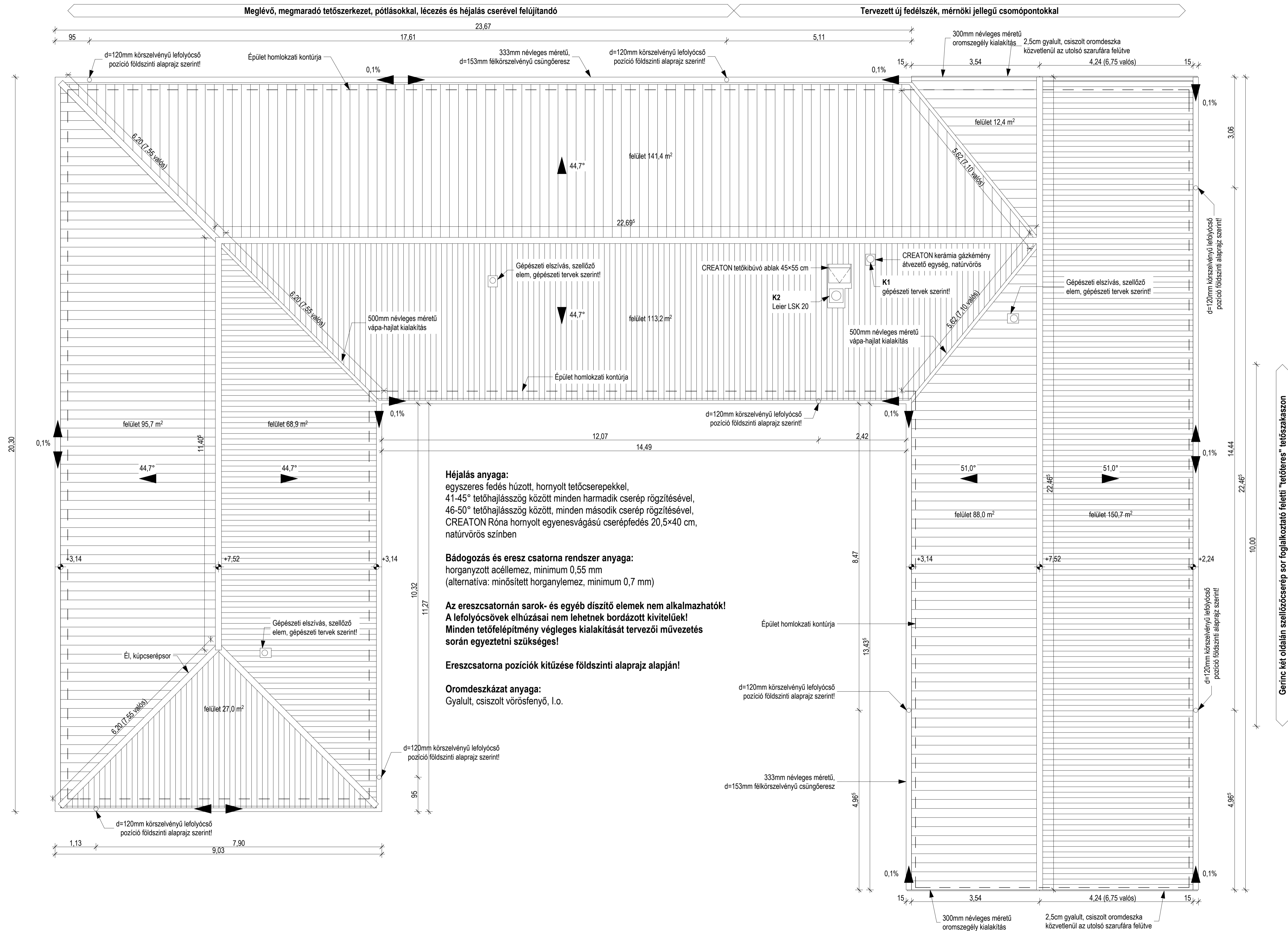
TETŐ ALAPRAJZA M=1:50
