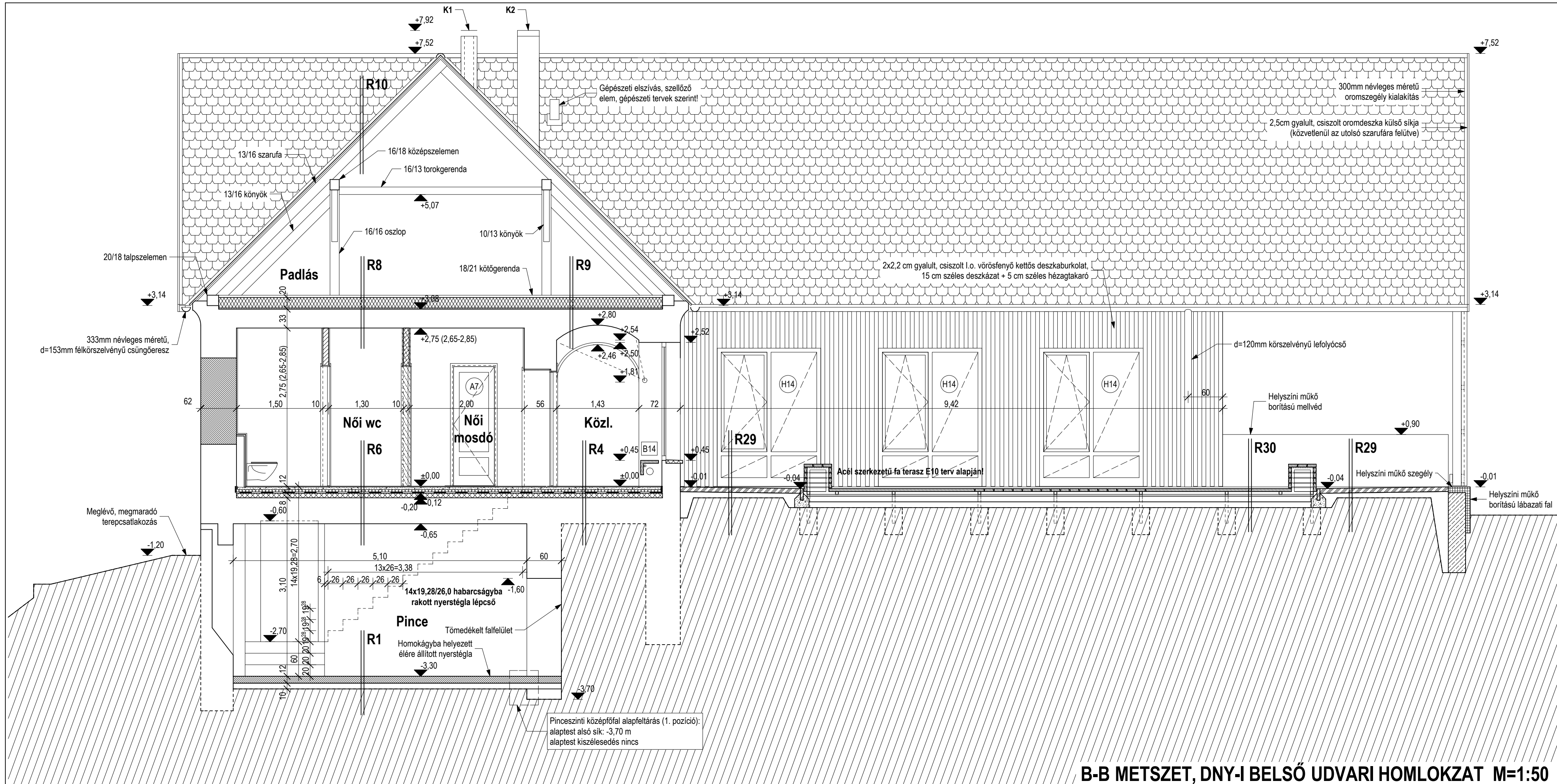
B-B METSZET, DNY-I BELSŐ UDVARI HOMLOKZAT M=1:50
