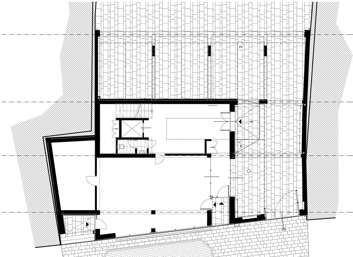
Földszinti alaprajz
