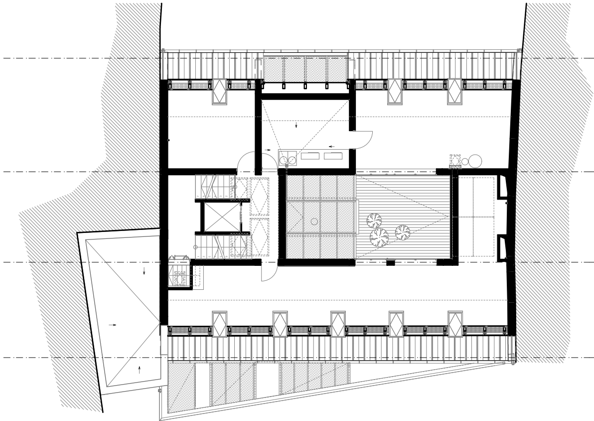
Tetőtéri alaprajz
