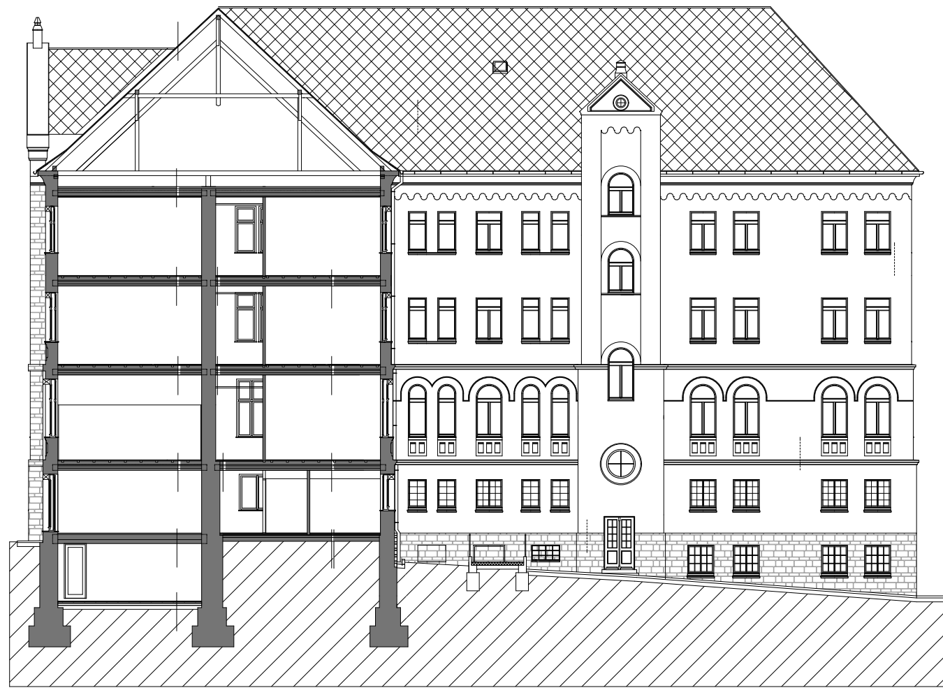
Tervezett A-A metszet m 1:100
