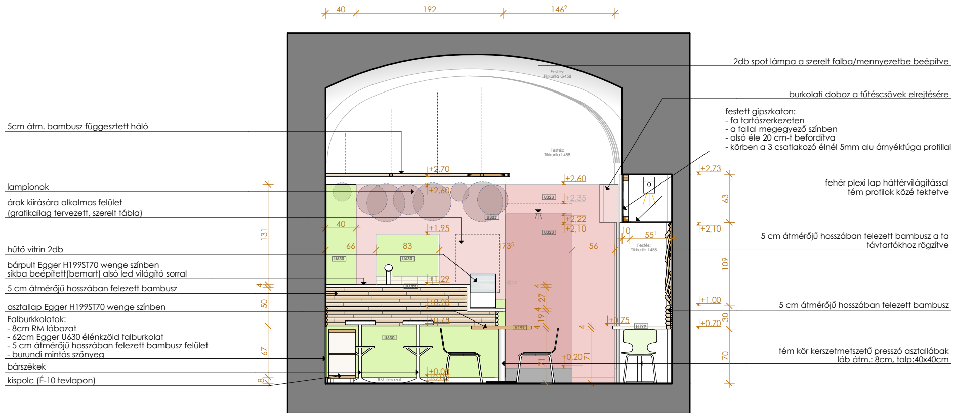
B metszet m1:50
