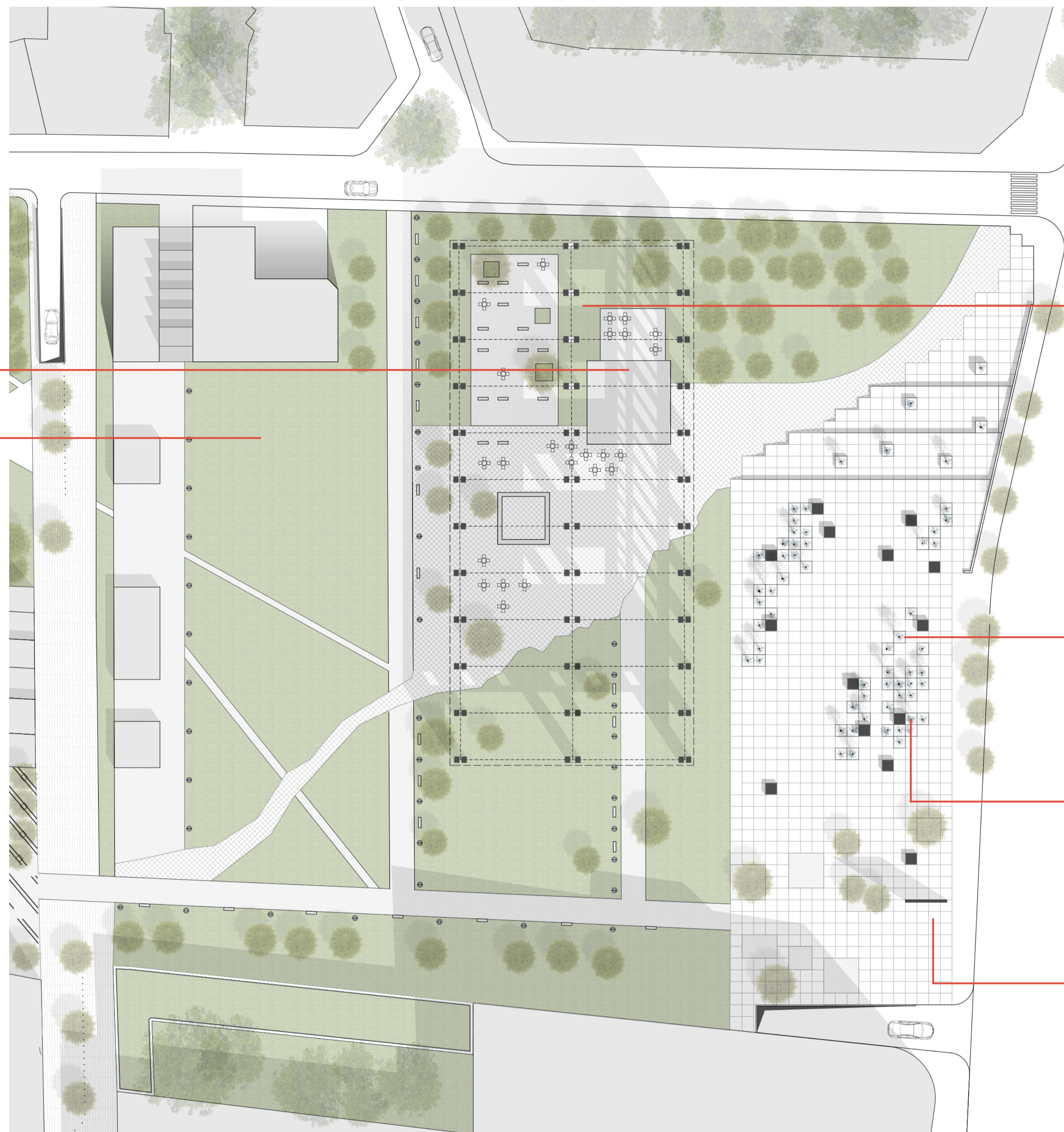
1.1. Helyszínrajz 1:500
