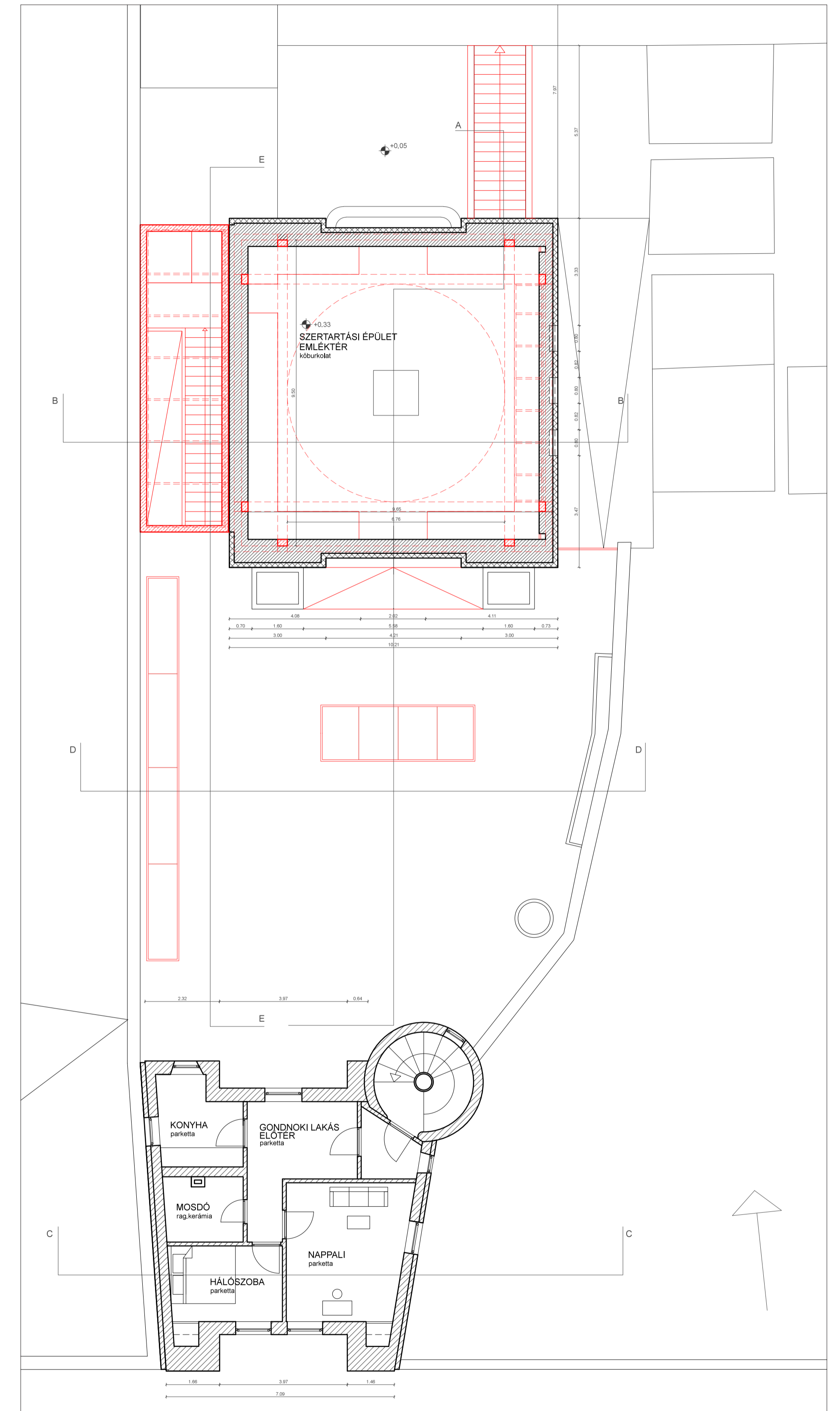
EMELETI ALAPRAJZ
