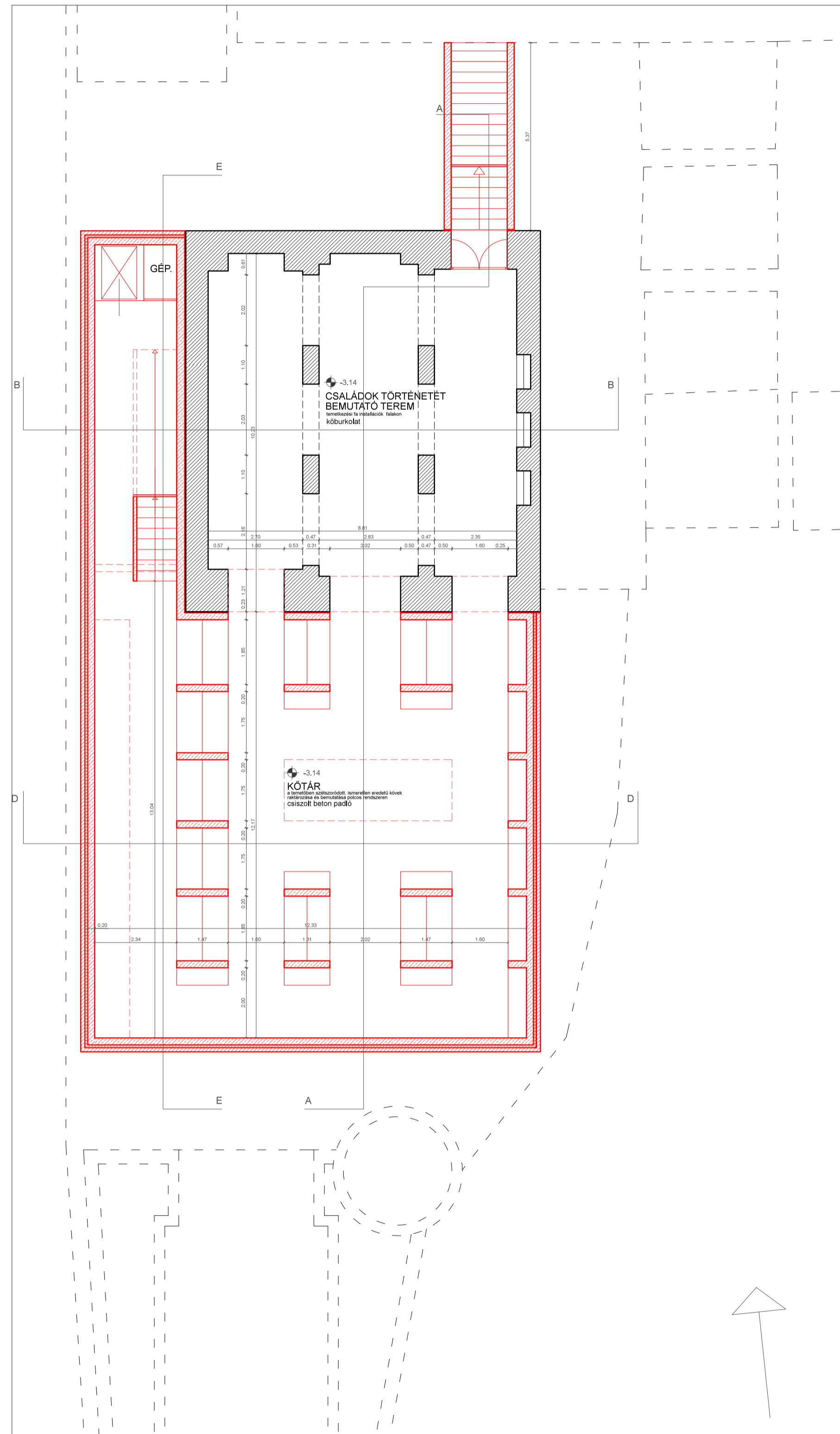
PINCESZINTI ALAPRAJZ
