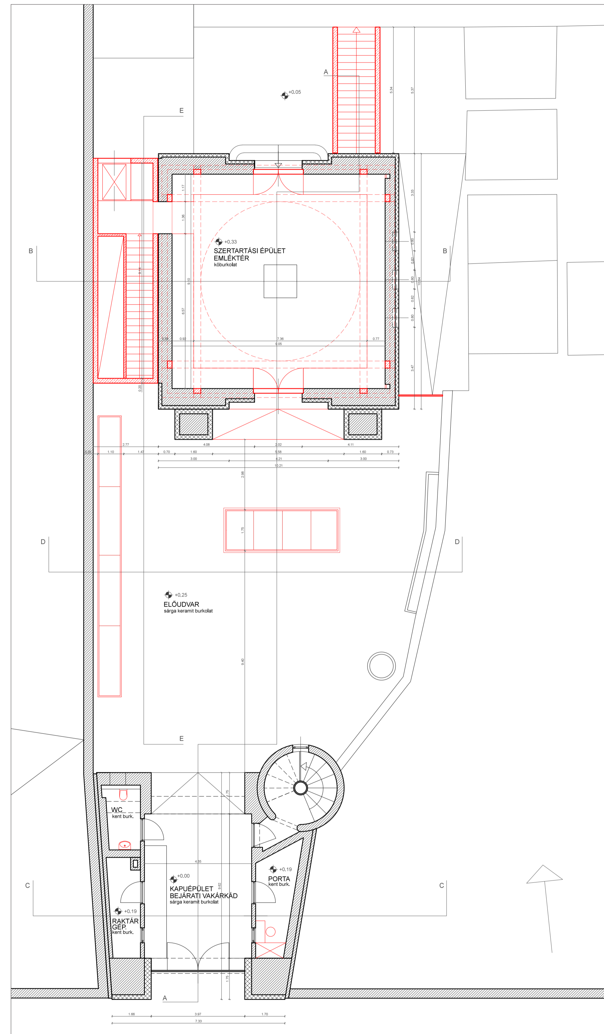
FÖLDSZINTI ALAPRAJZ
