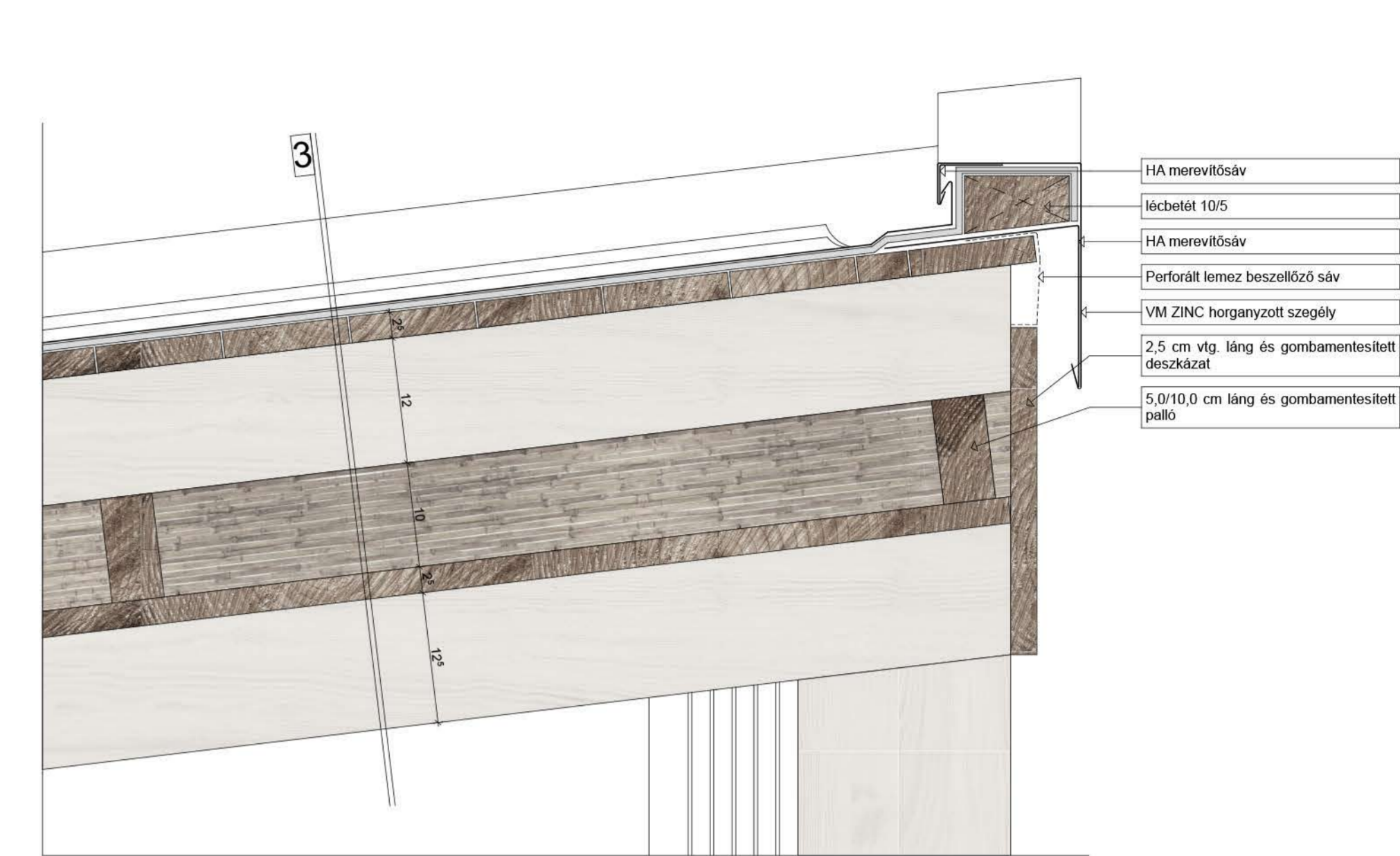
10 OROMSZEGÉLY RÉSZLETRAJZA M=1:5
