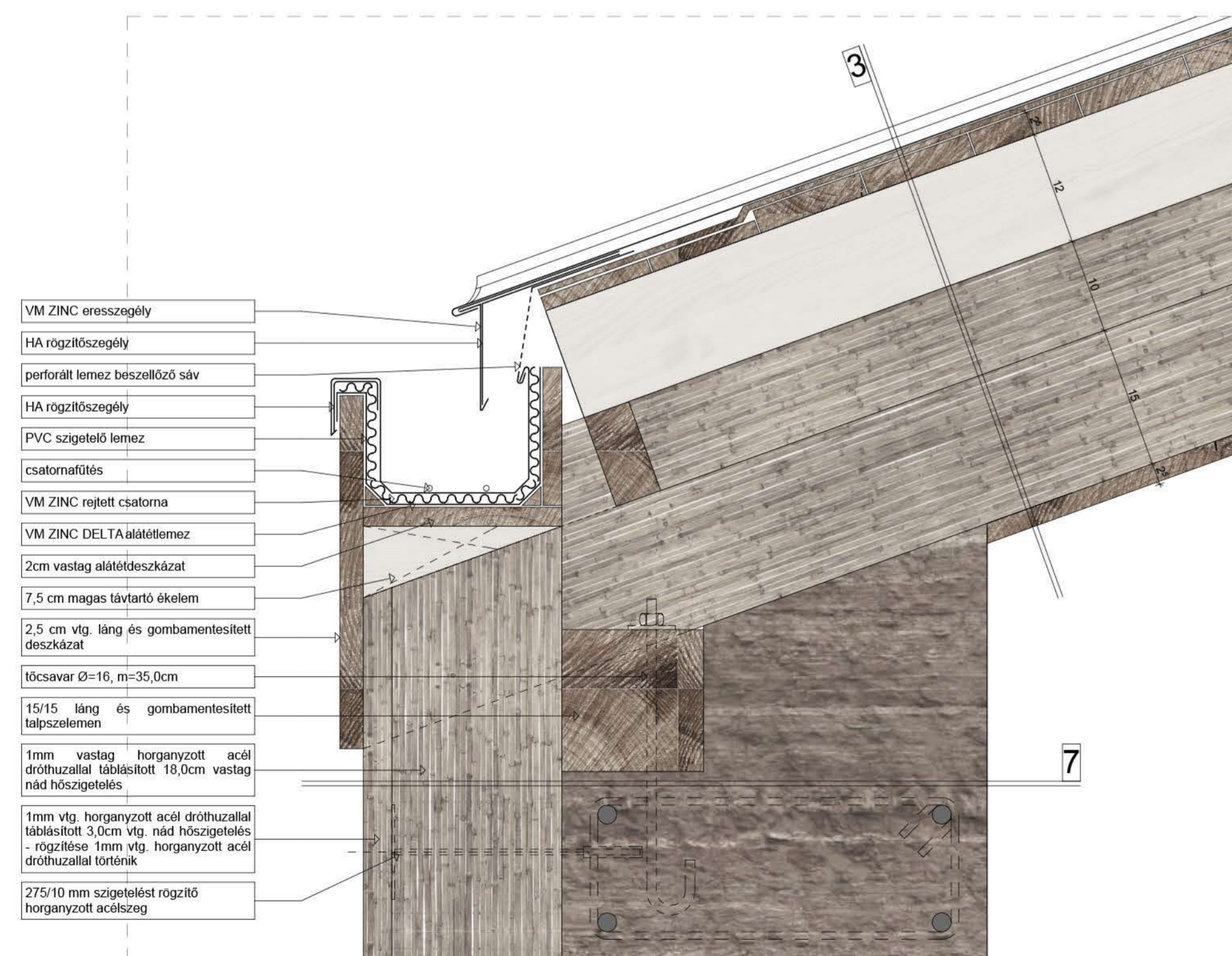
7 REJTETT ERESZ RÉSZLETRAJZA M=1:5
