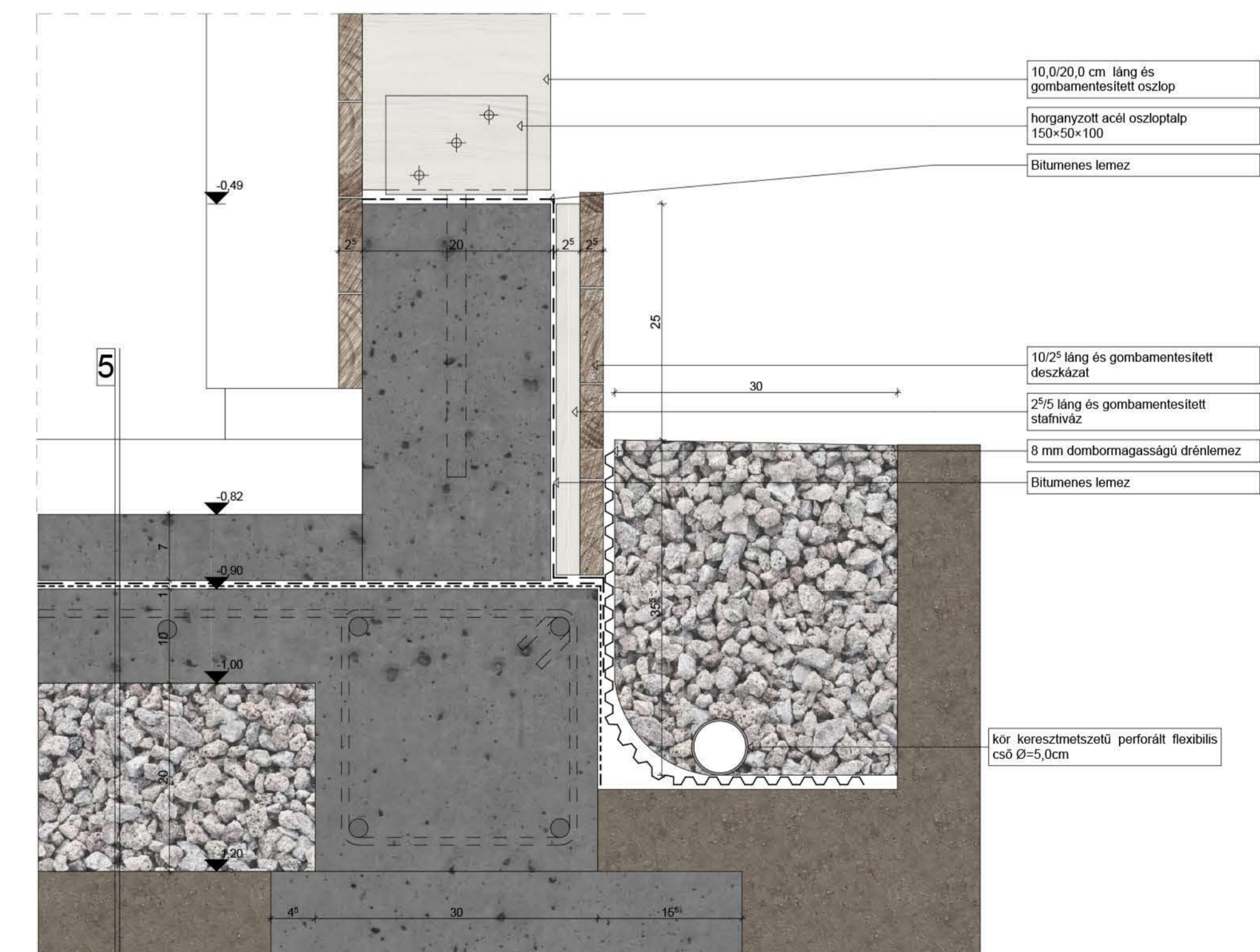
10 LÁBAZAT RÉSZLETRAJZA M=1:5
