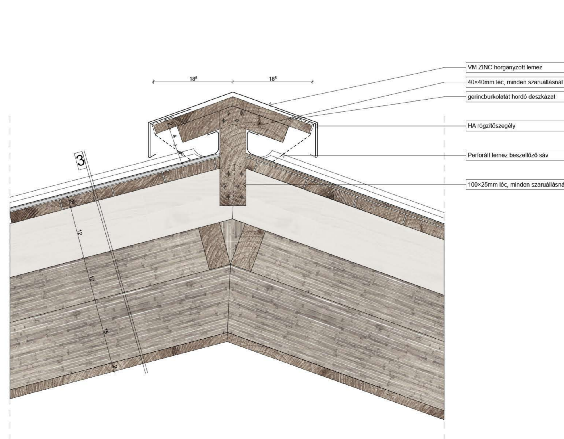
9 TETŐGERINC RÉSZLETRAJZA M=1:5
