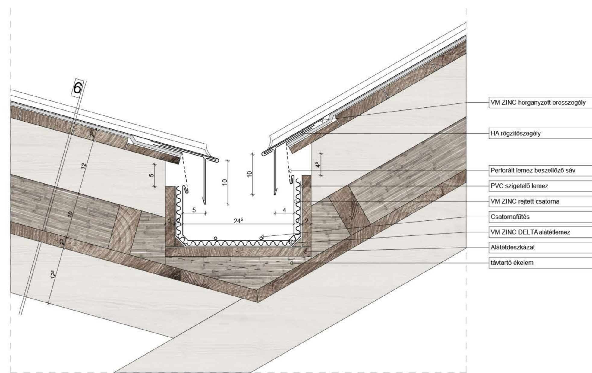
10 VÁPACSATORNA RÉSZLETRAJZA M=1:5
