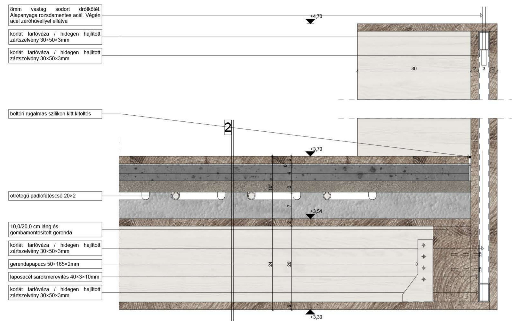
8 KORLÁT RÉSZLETRAJZA M=1:5
