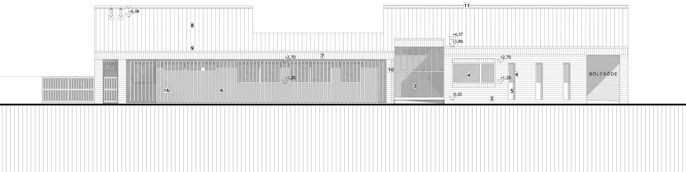
ÉSZAKNYUGATI HOMLOKZAT M=1:100
