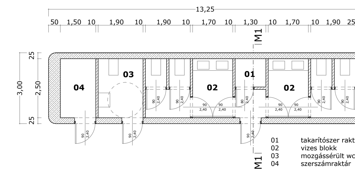
Melléképület alaprajz M = 1 : 100
