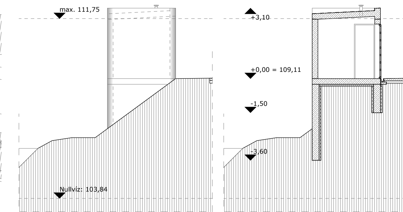
Nyugati homlokzat M = 1 : 100
