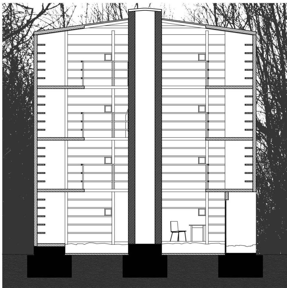
metszet m 1:100
