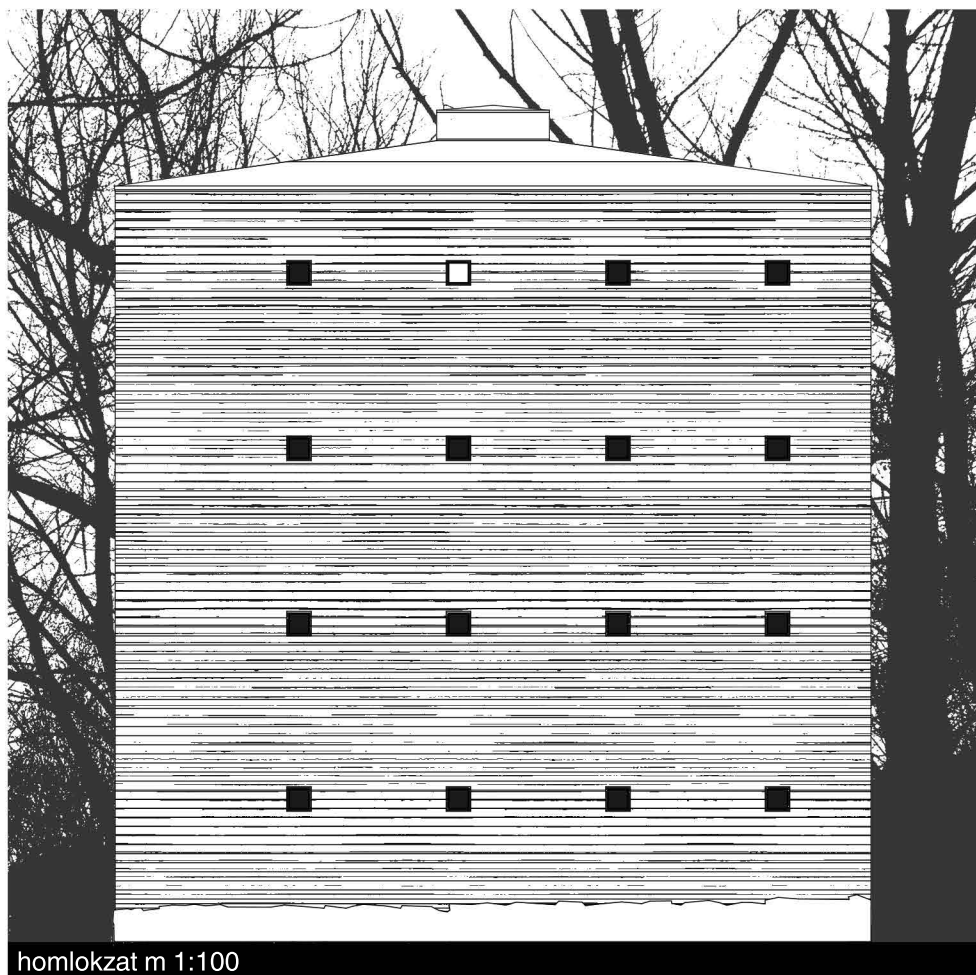
homlokzat m 1:100
