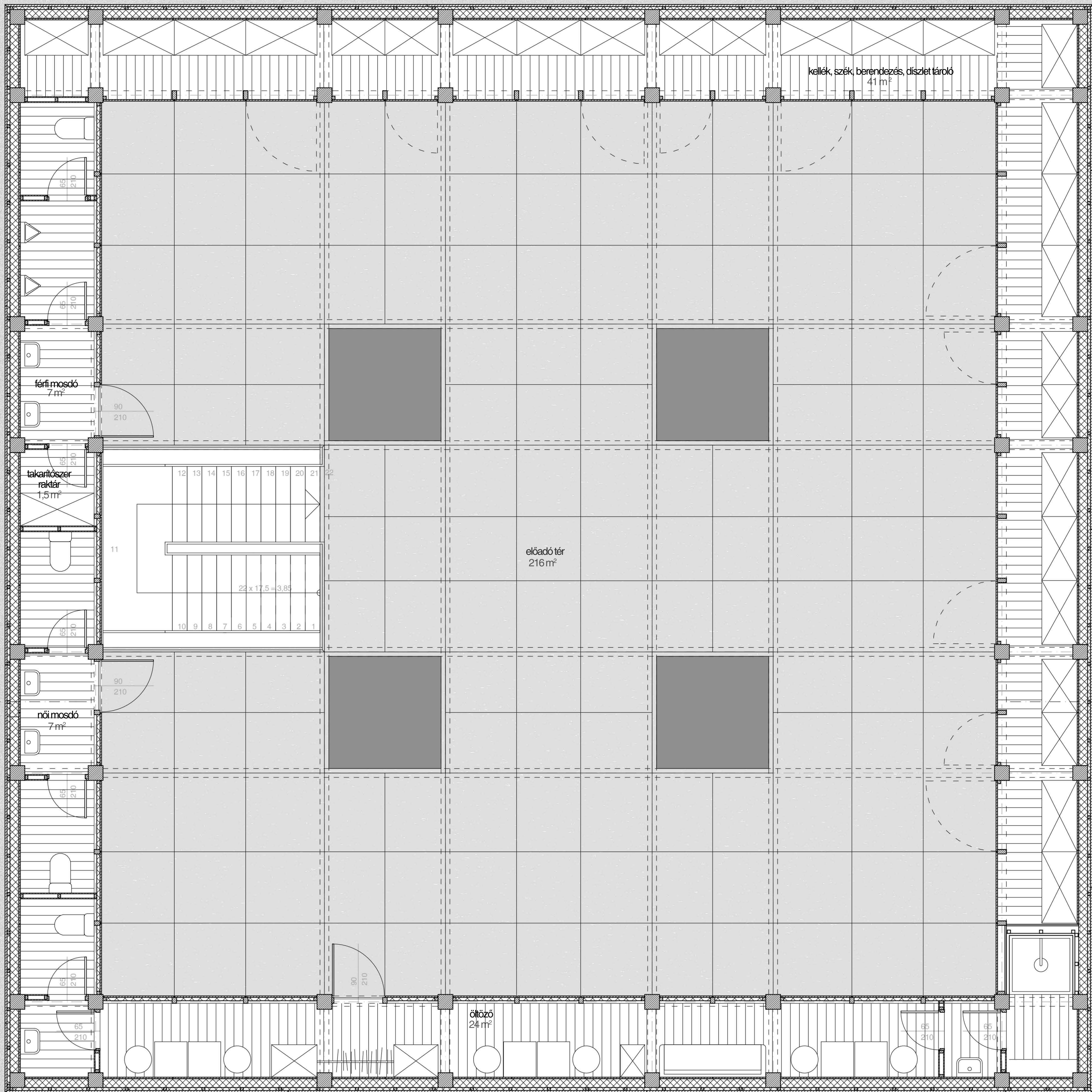
emeleti alaprajz M 1:50
