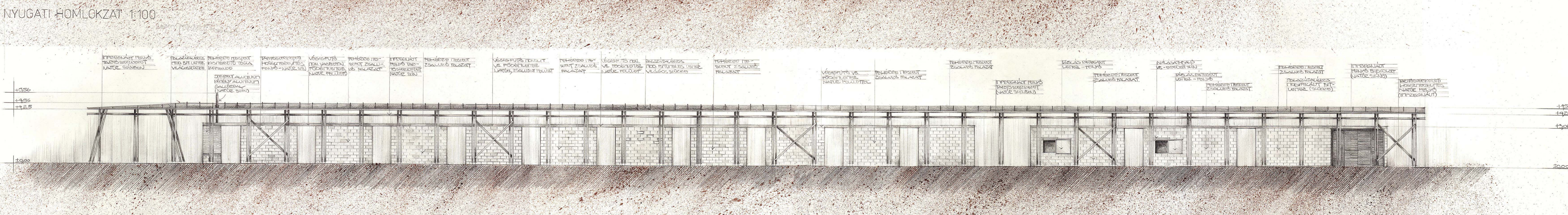
KELETI HOMLOKZAT 1:100
