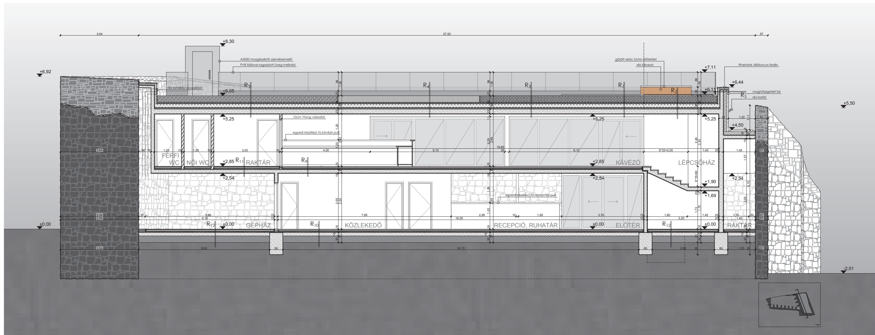
A-A METSZET
