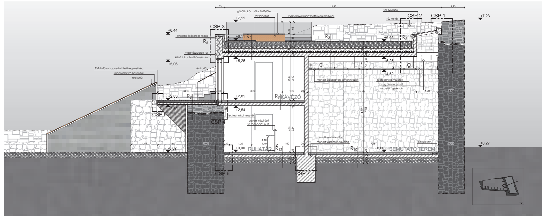
B-B METSZET
