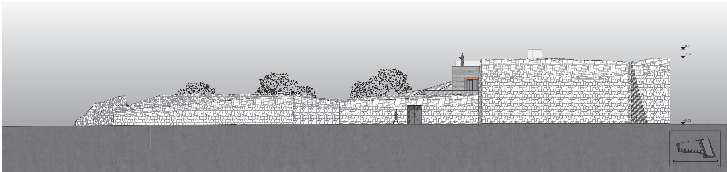
KELETI HOMLOKZAT
