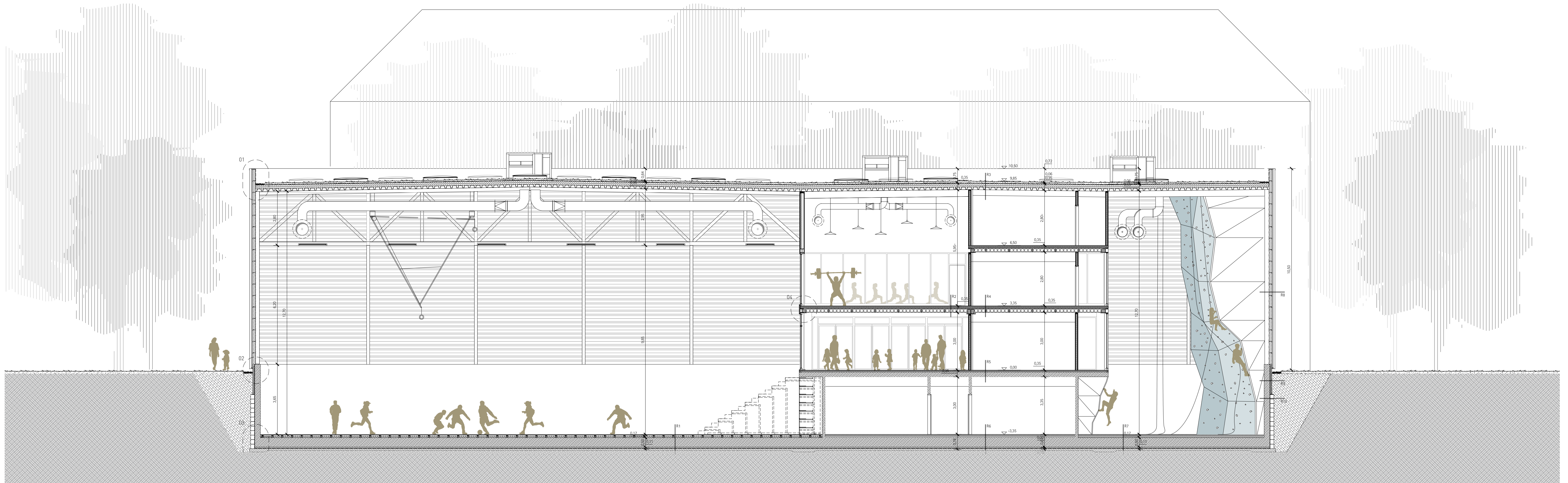
Keresztmetszet
