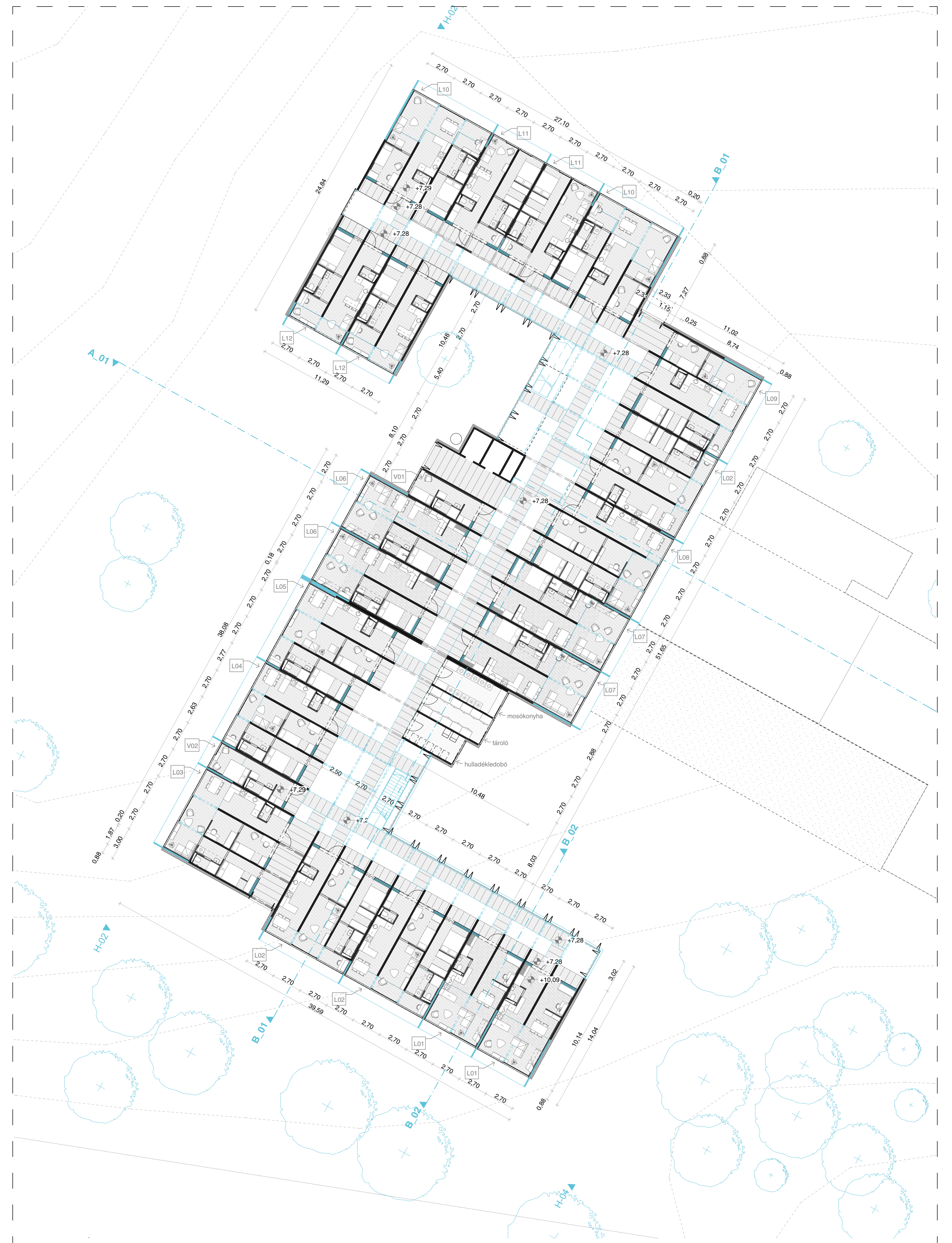
1., 3. emeleti alaprajz M=1:200
