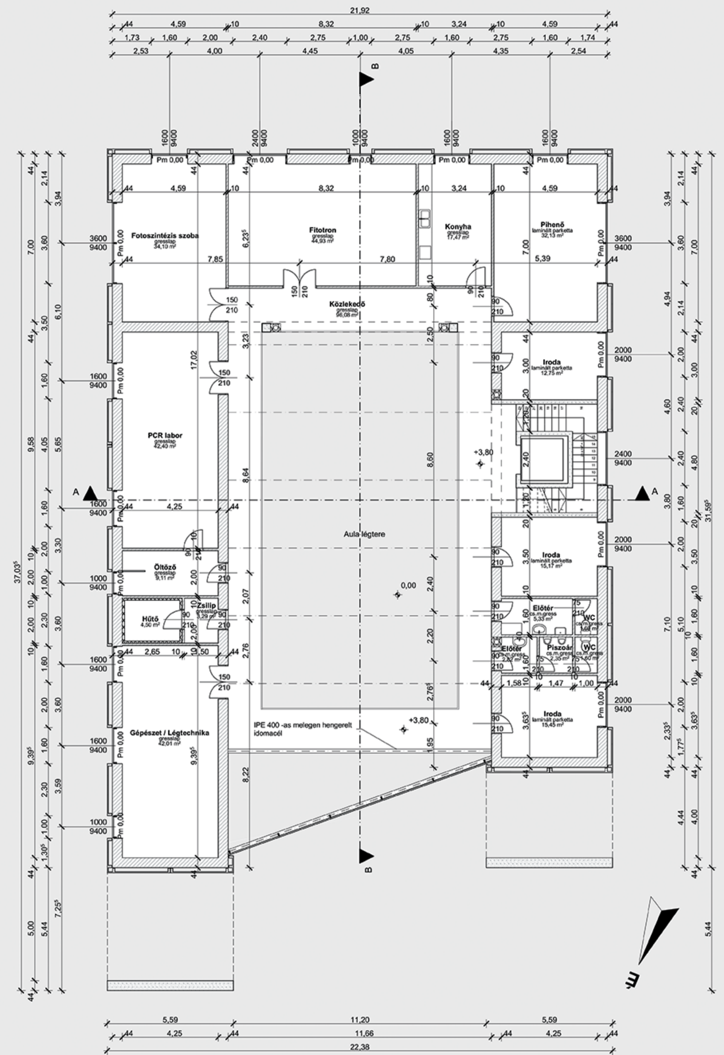
EMELETI ALAPRAJZ M = 1:100
