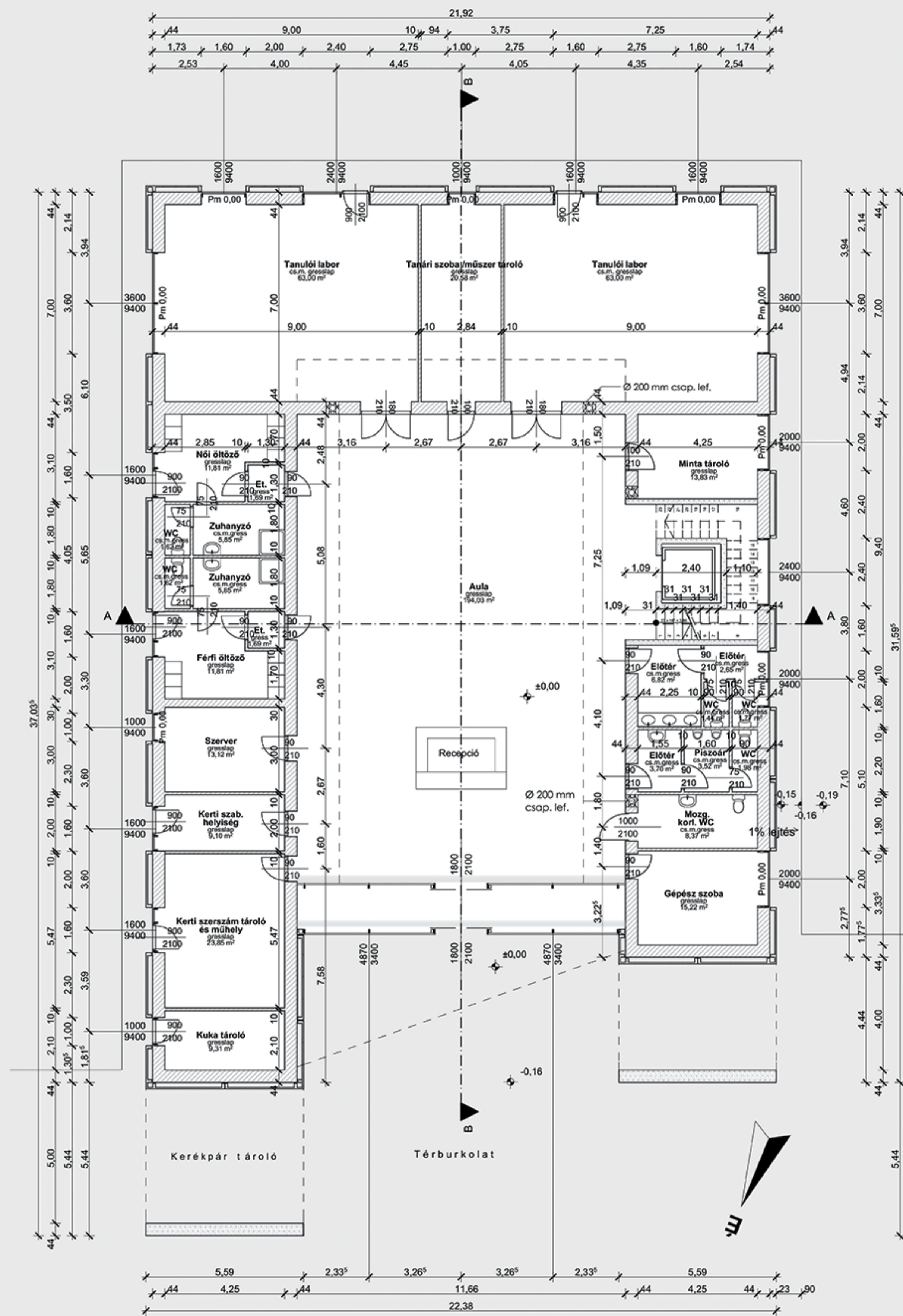
FÖLDSZINTI ALAPRAJZ M = 1:100
