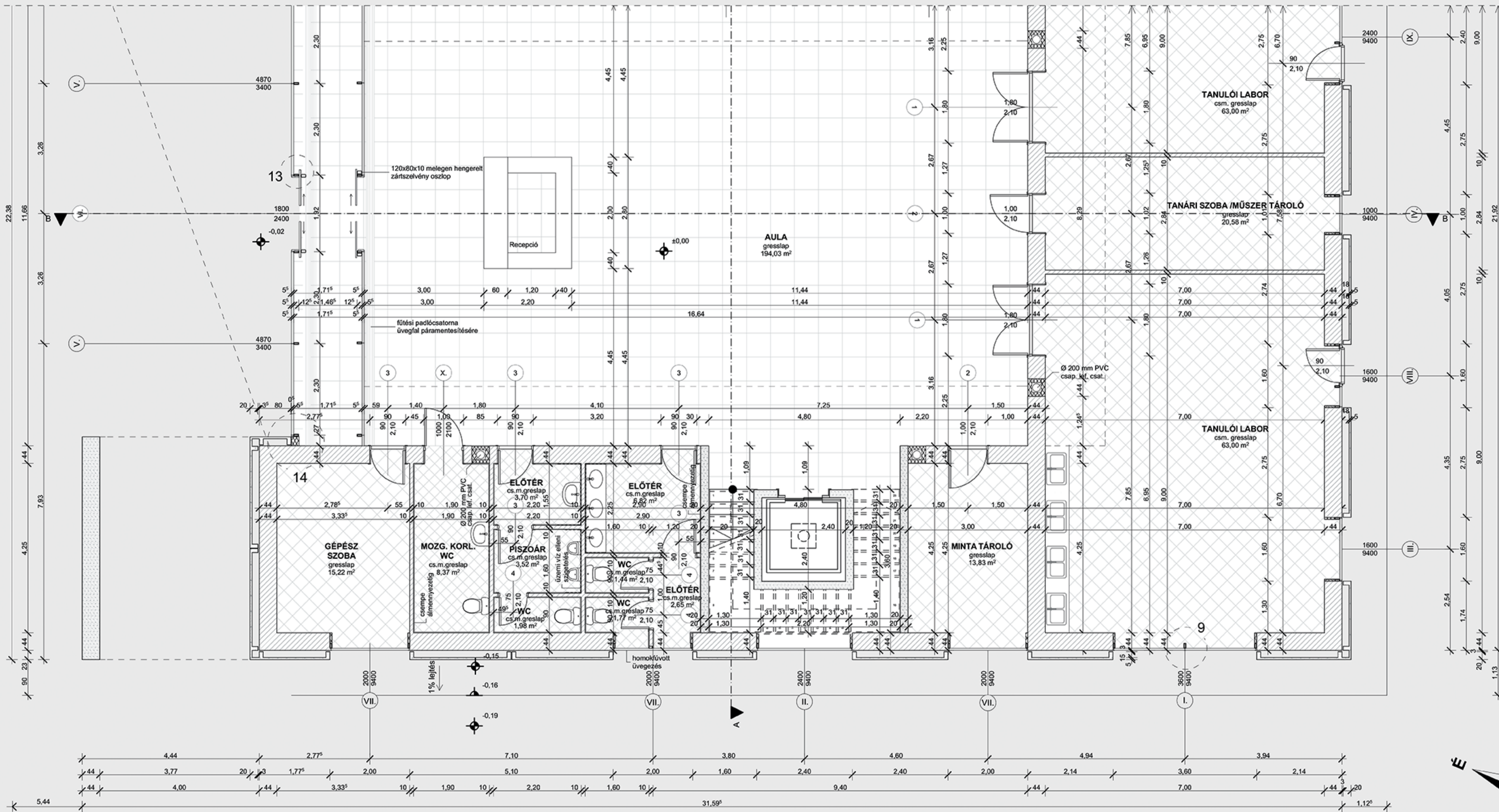
Földszinti alaprajzi részlet M = 1:50
