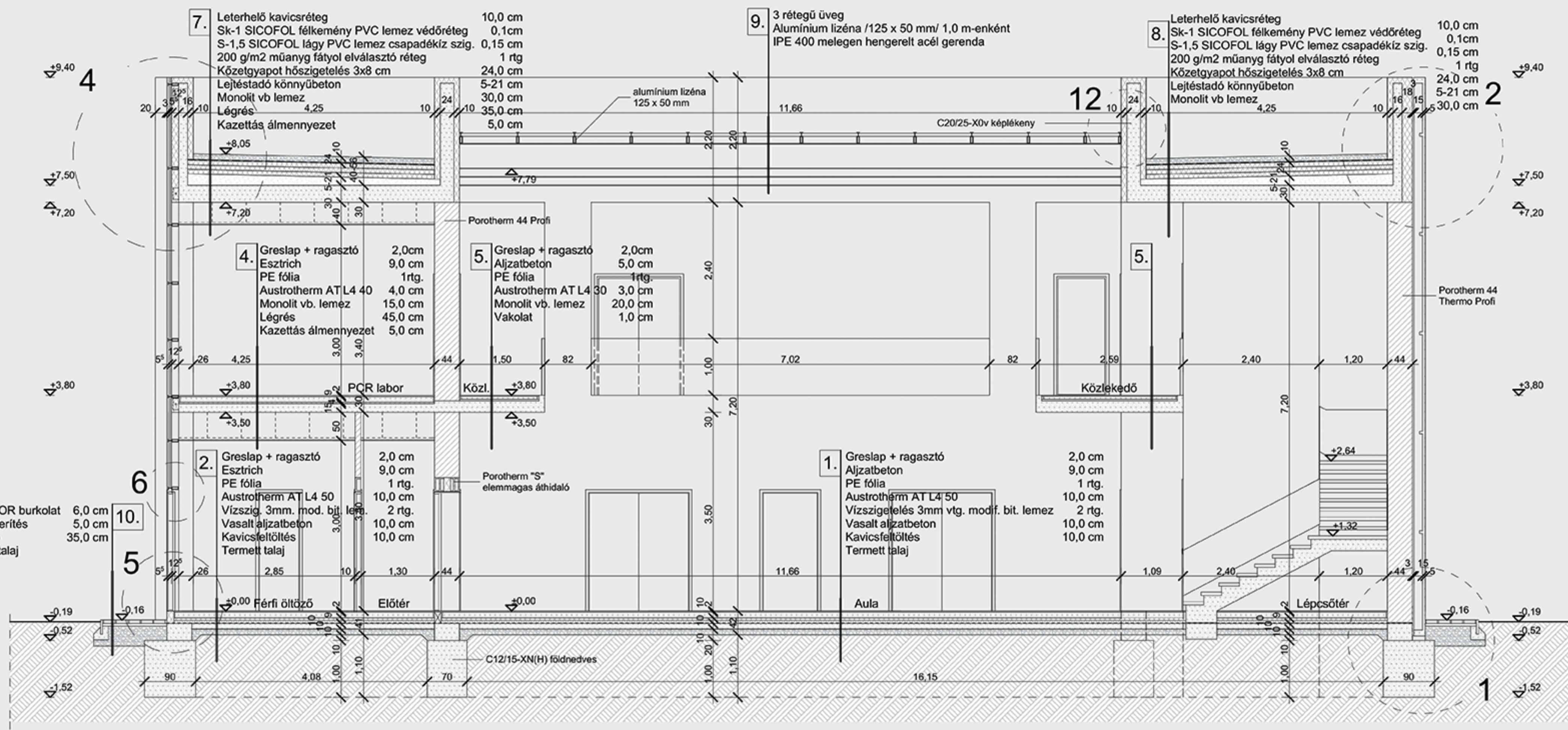
A - A metszet M = 1:50
