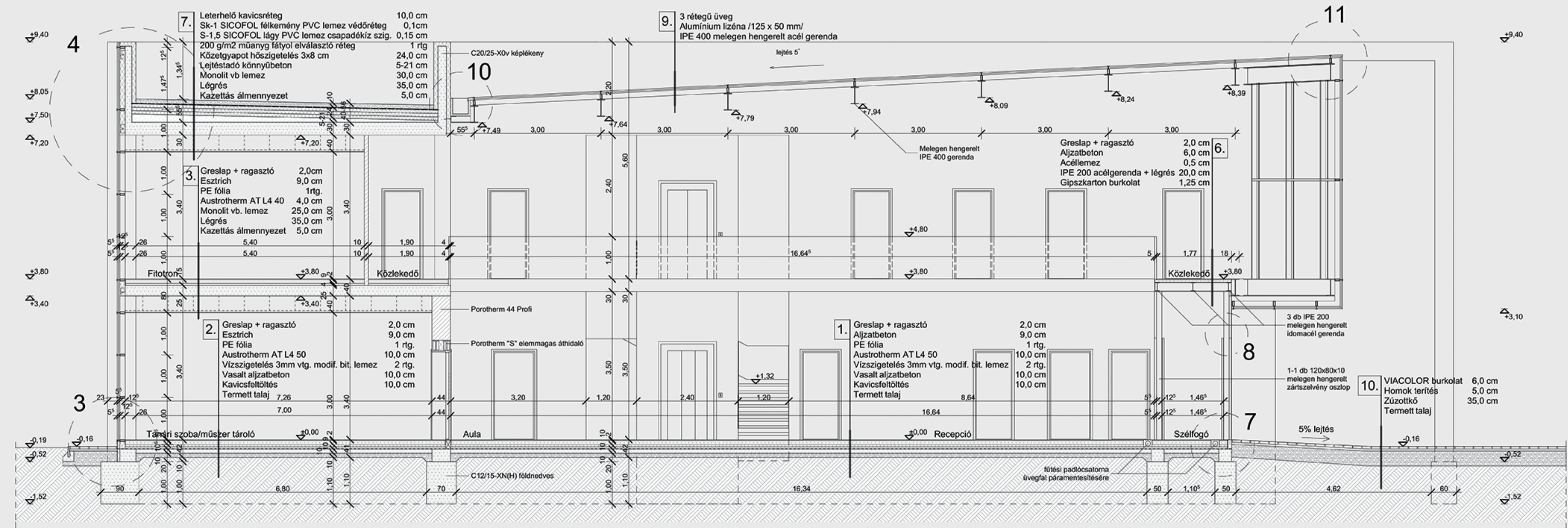
B - B metszet M = 1:50
