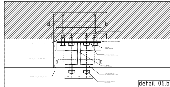
detail 06.a
