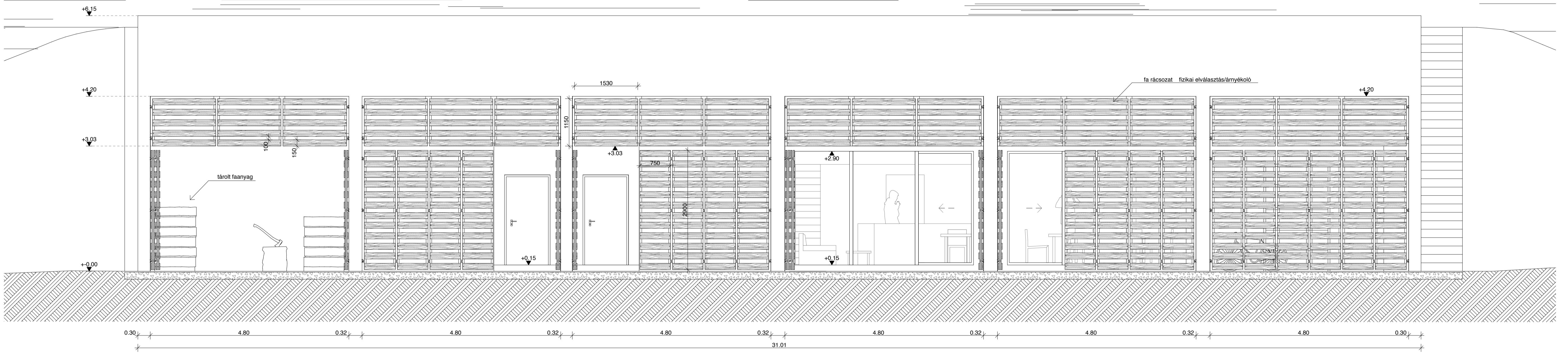
1.sz. Bunker / homlokzat M=1:50
