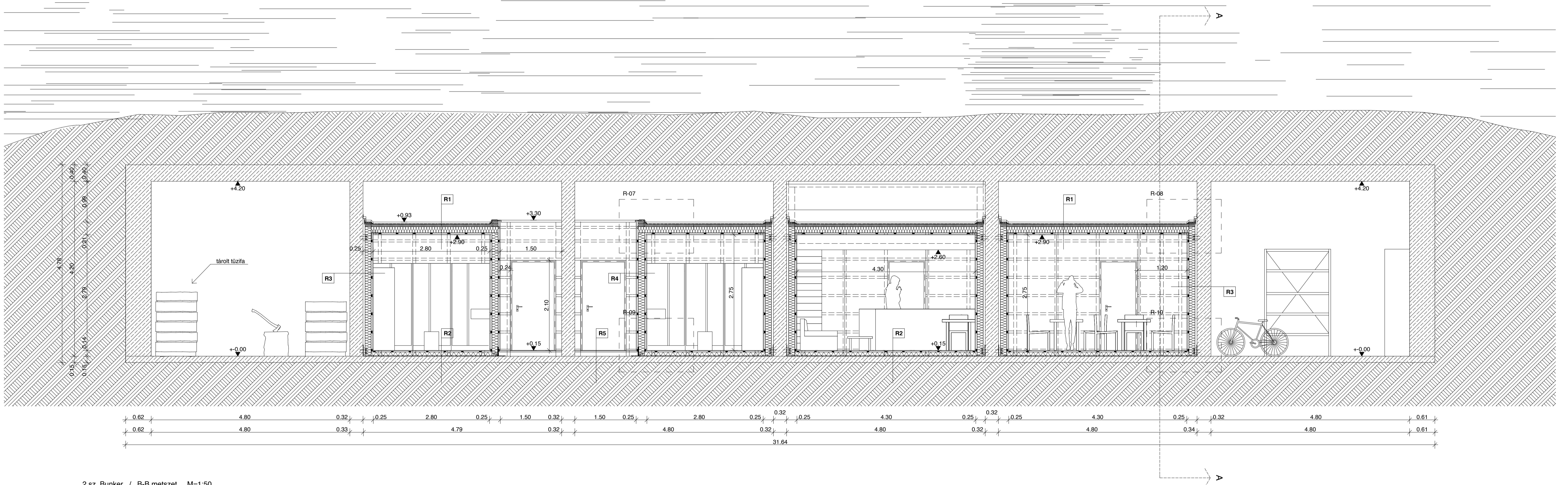
2.sz. Bunker / B-B metszet M=1:50
