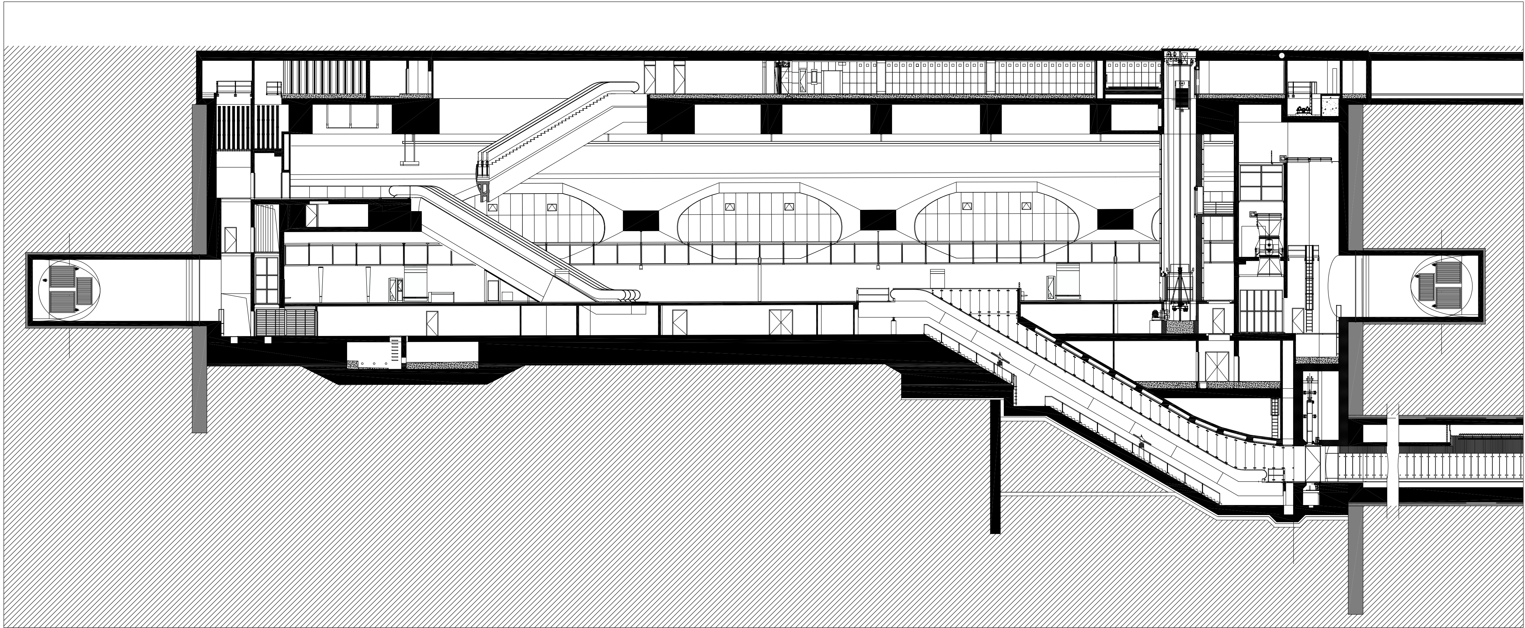
longitudinal section
