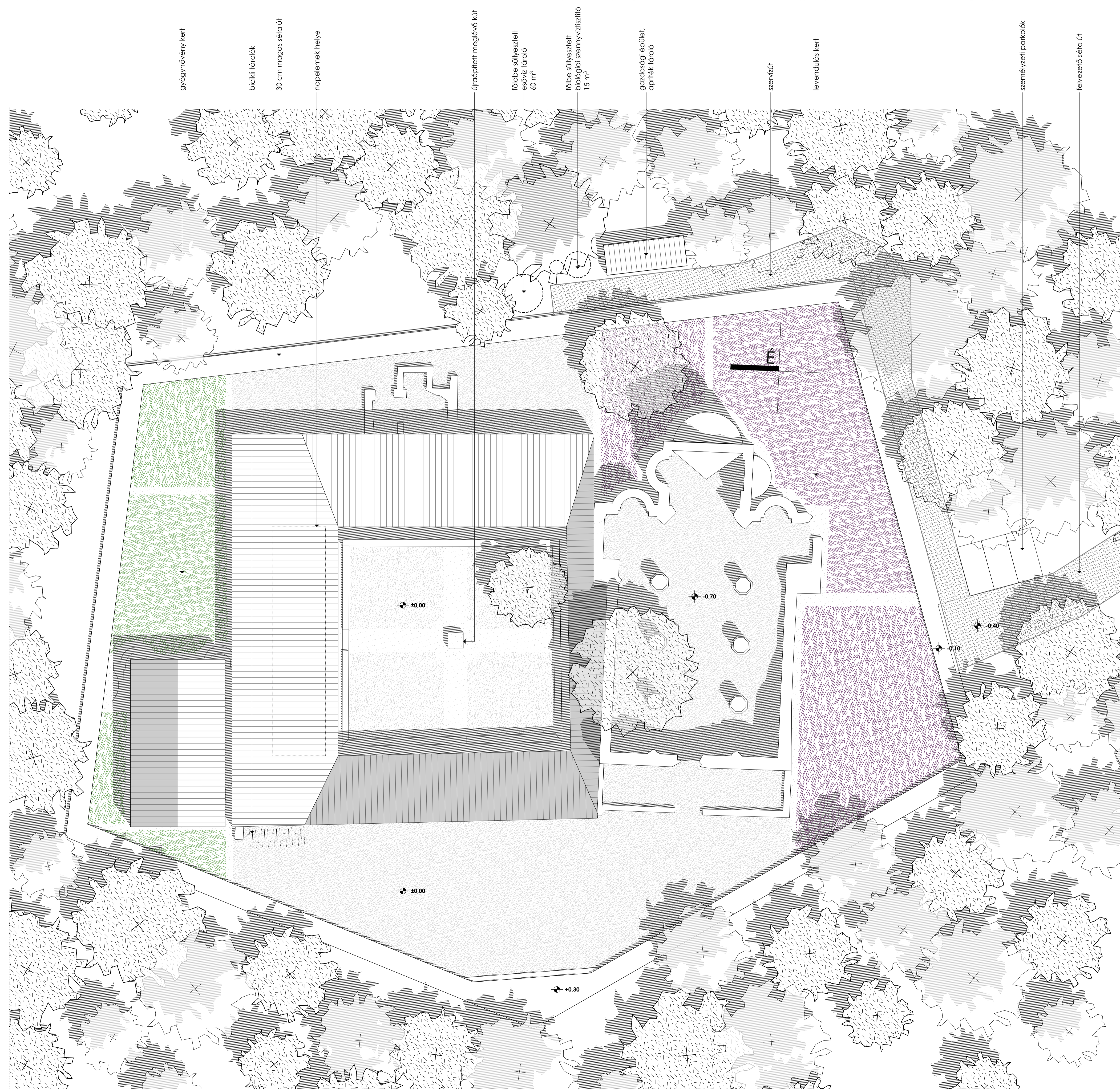
helyszínrajz m 1:500
