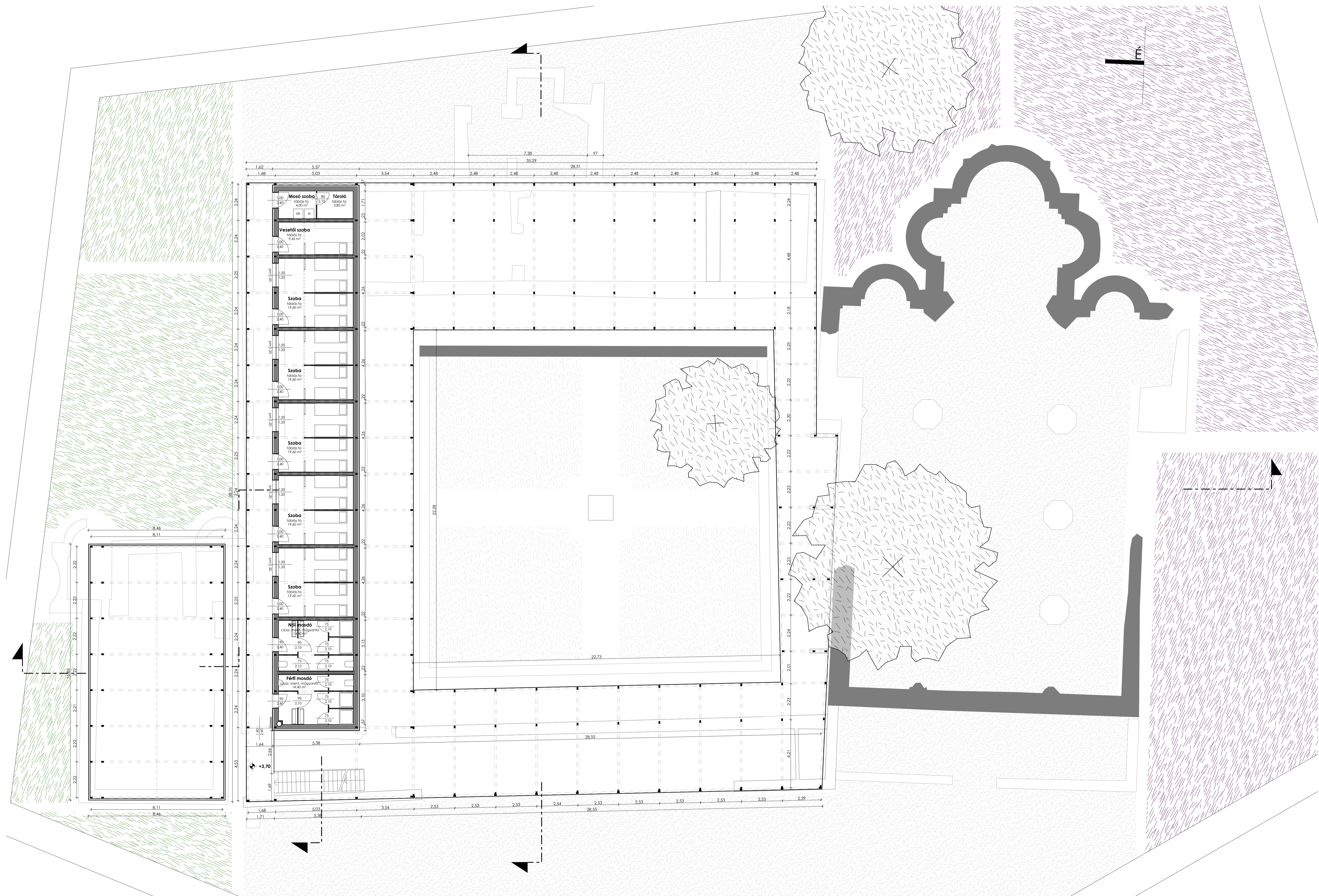
emeleti alaprajz m 1:100
