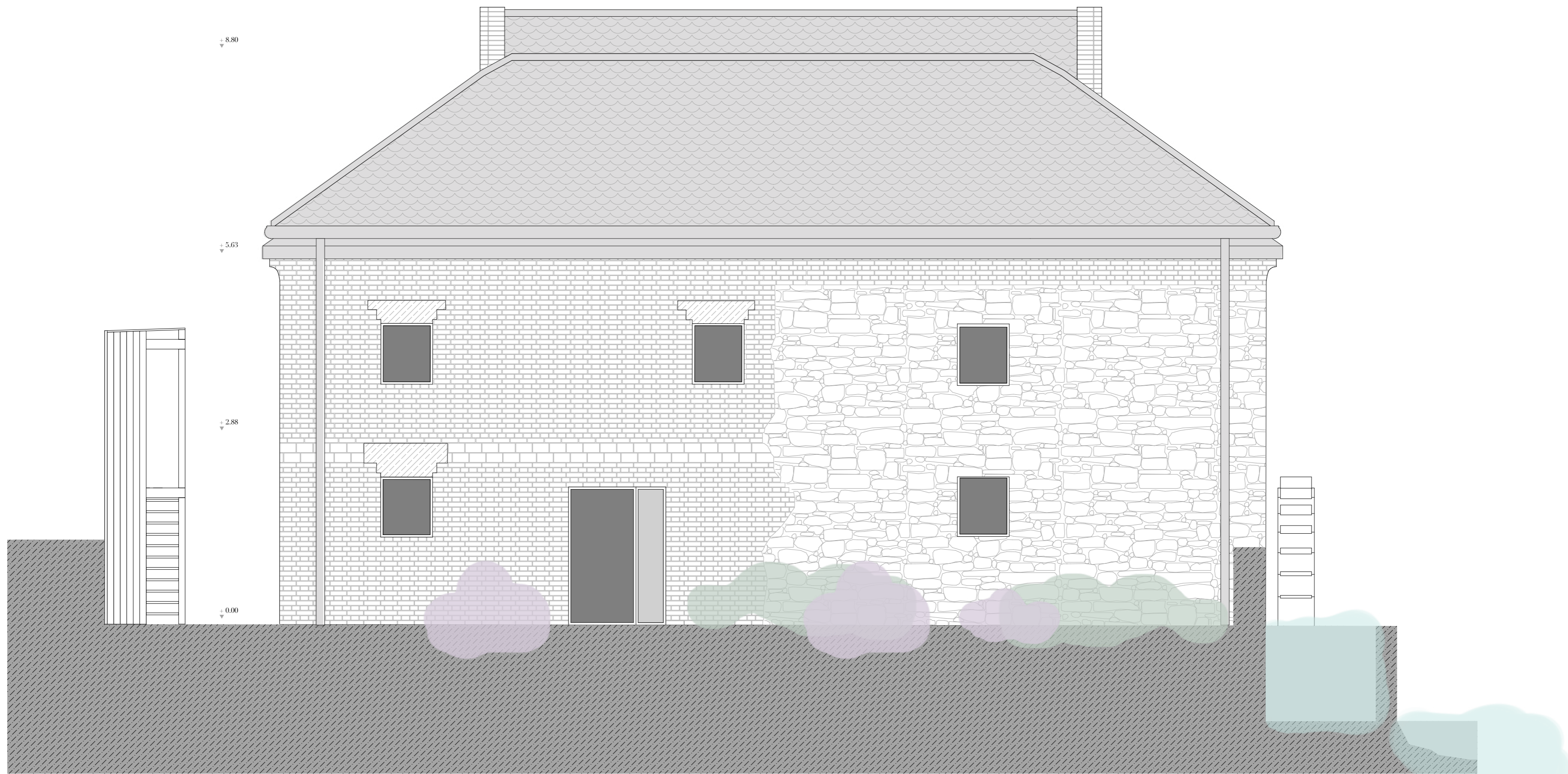
északi homlokzat m 1:50
