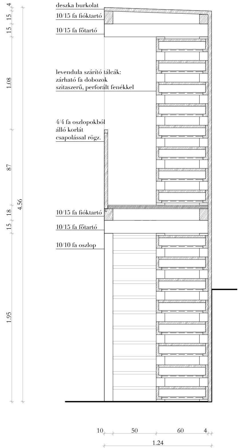
CSP8 - levendula szárító részletrajza m 1:10
