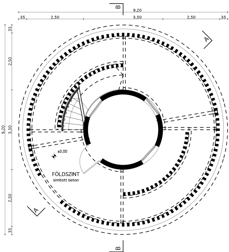
FÖLDSZINTI ALAPRAJZ
