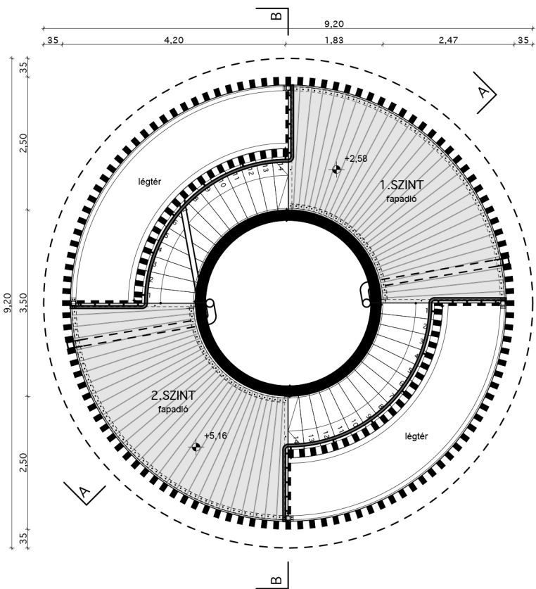
1.-2. SZINTI ALAPRAJZ
