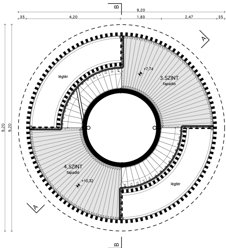
3.-4. SZINTI ALAPRAJZ
