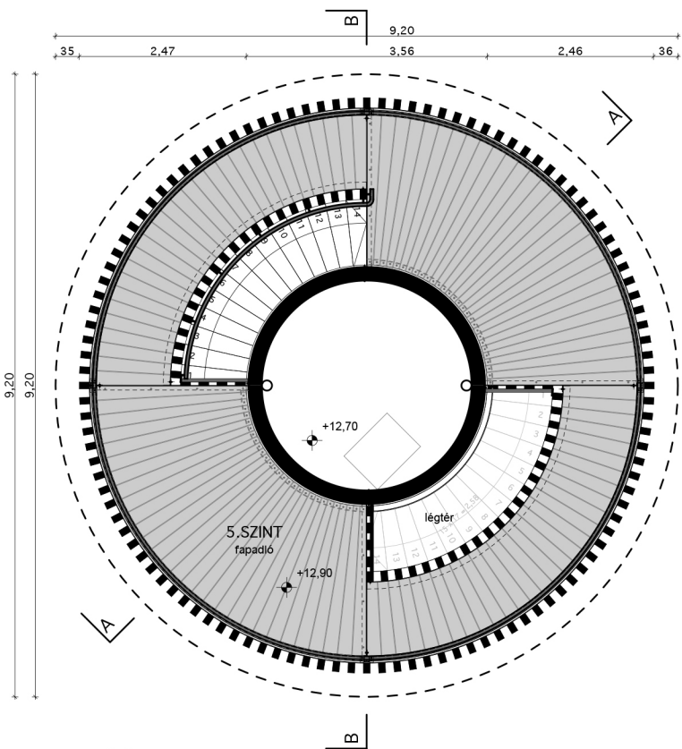
KILÁTÓ SZINTI ALAPRAJZ
